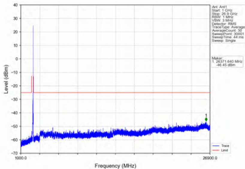
n41 30kHz SISO NTV 40MHz DFT-s-OFDM QPSK 2516.01MHz Edge 1RB Left
