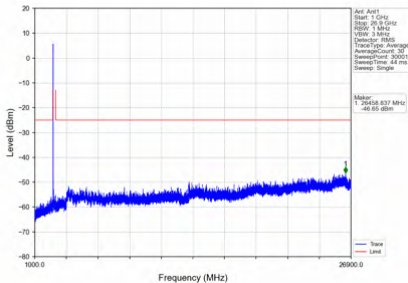
n41_30kHz_SISO_NTNV_20MHz_CP-OFDM QPSK_2592.99MHz_Edge_1RB_Left
