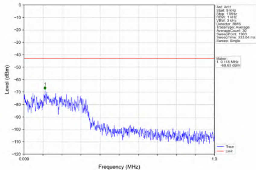
n41_30kHz_SISO_NTNV_20MHz_DFT-s-OFDM QPSK_2506.02MHz_Edge_1RB_Left
