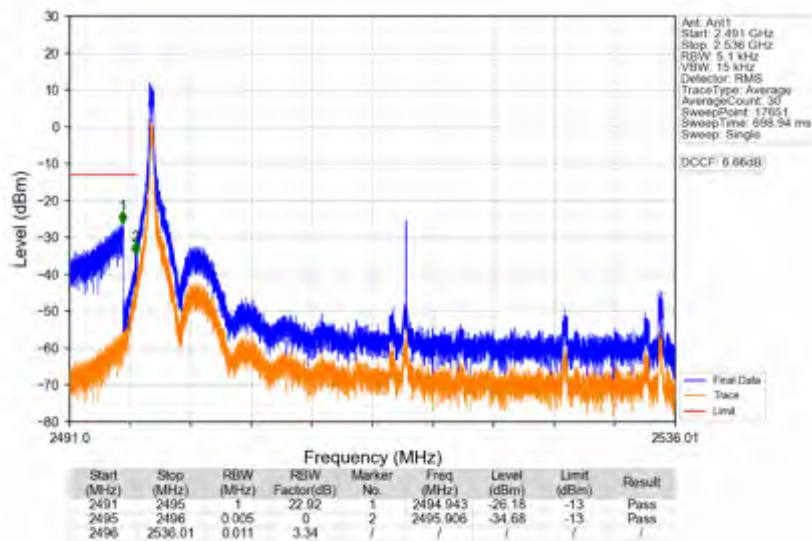
n41 30kHz SISO NTV 40MHz DFT-s-OFDM QPSK 2516.01MHz Edge 1RB Left
