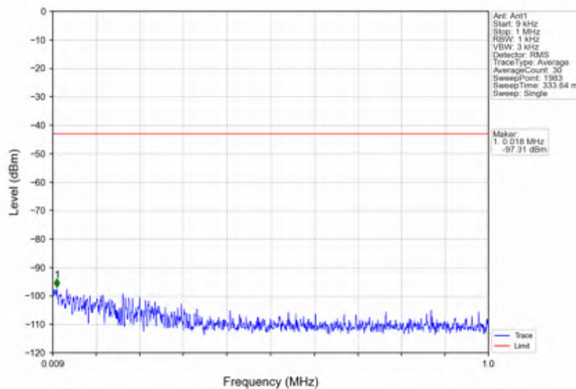
n41_30kHz_SISO_NTNV_40MHz_CP-OFDM QPSK_2670MHz_Inner_1RB_Right
