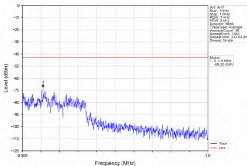
n41_30kHz_SISO_NTNV_20MHz_DFT-s-OFDM_PI/2_BPSK_2506.02MHz_Edge_1RB_Left
