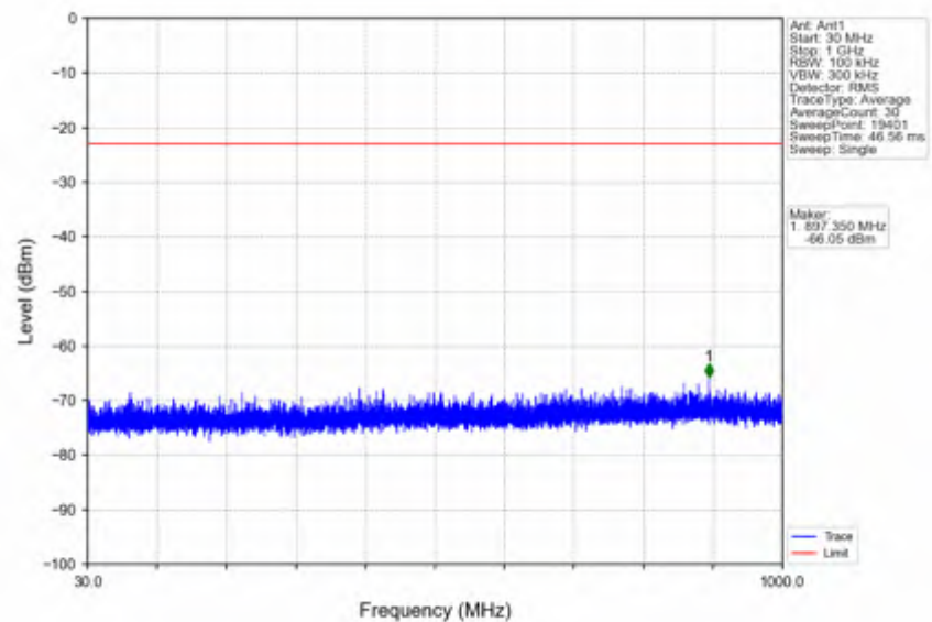
n41_30kHz_SISO_NTNV_30MHz_CP-OFDM_QPSK_2511MHz_Inner_1RB_Left
