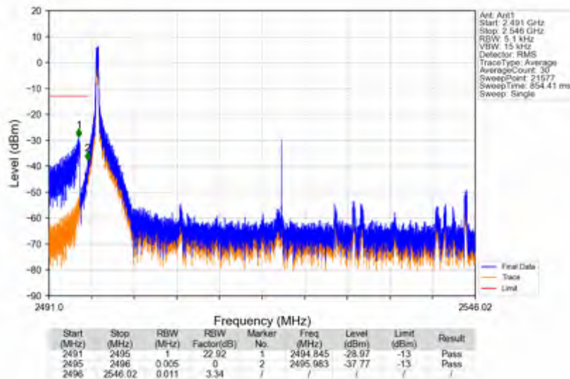
n41_30kHz_SISO_NTNV_50MHz_DFT-s-OFDM_PI/2_BPSK_2521.02MHz_Edge_1RB_Left
