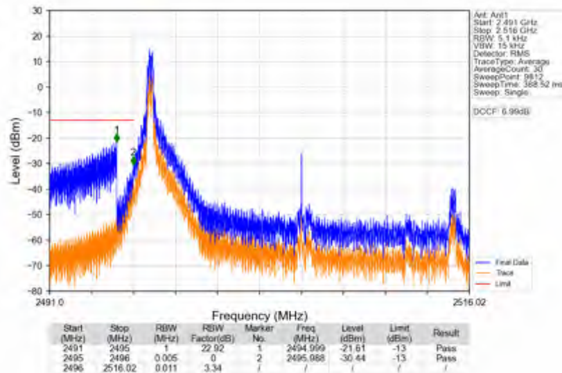
n41_30kHz_SISO_NTNV_20MHz_DFT-s-OFDM_PI/2_BPSK_2506.02MHz_Edge_1RB_Left
