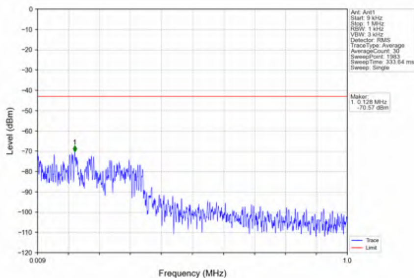
n41_30kHz_SISO_NTNV_50MHz_DFT-s-OFDM_PI/2_BPSK_2521.02MHz_Edge_1RB_Left
