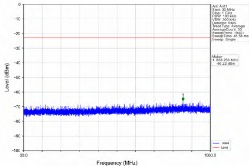
n41_30kHz_SISO_NTNV_40MHz_DFT-s-OFDM QPSK_2670MHz_Inner_1RB_Right
