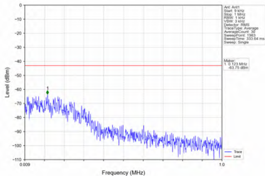
n41_30kHz_SISO_NTNV_20MHz_CP-OFDM QPSK_2592.99MHz_Edge_1RB_Left
