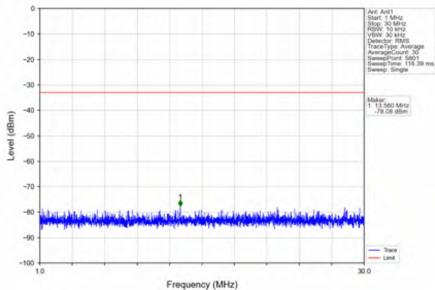
n41_30kHz_SISO_NTNV_20MHz_CP-OFDM QPSK_2679.99MHz_Inner_1RB_Right
