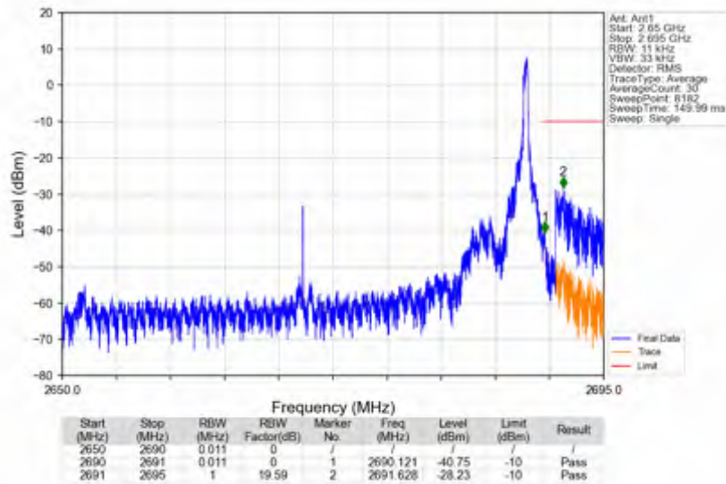
n41_30kHz_SISO_NTNV_40MHz_CP-OFDM QPSK_2670MHz_Inner_1RB_Right
