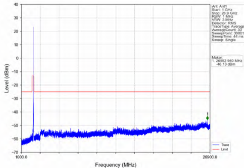
n41_30kHz_SISO_NTNV_40MHz_DFT-s-OFDM QPSK_2670MHz_Inner_1RB_Right
