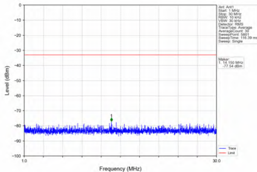
n41_30kHz_SISO_NTNV_40MHz_CP-OFDM QPSK_2670MHz_Inner_1RB_Right
