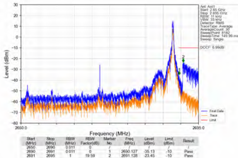
n41_30kHz_SISO_NTNV_40MHz_DFT-s-OFDM QPSK_2670MHz_Inner_1RB_Right
