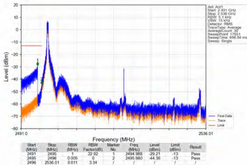
n41_30kHz_SISO_NTNV_40MHz_DFT-s-OFDM QPSK_2516.01MHz_Inner_1RB_Left
