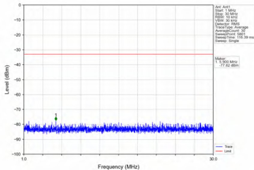
n41_30kHz_SISO_NTV_15MHz_CP-OFDM QPSK_2503.5MHz_Inner_1RB_Left
