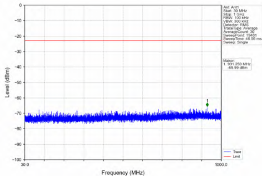
n41_30kHz_SISO_NTV_15MHz_CP-OFDM QPSK_2503.5MHz_Inner_1RB_Left
