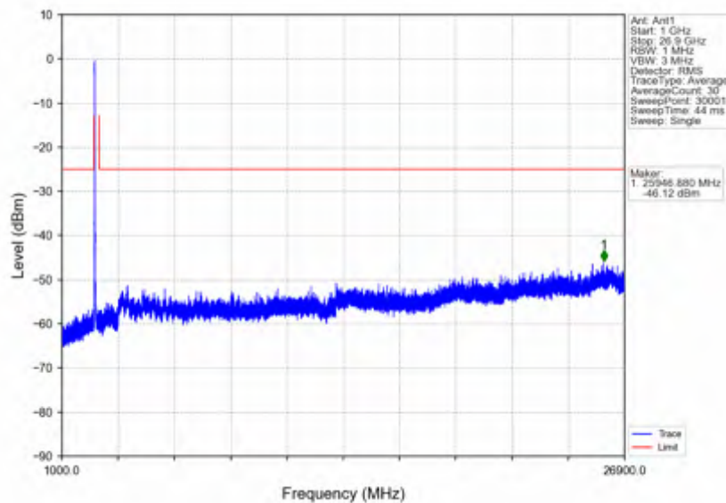
n41_30kHz_SISO_NTNV_20MHz_DFT-s-OFDM QPSK_2506.02MHz_Inner_1RB_Left
