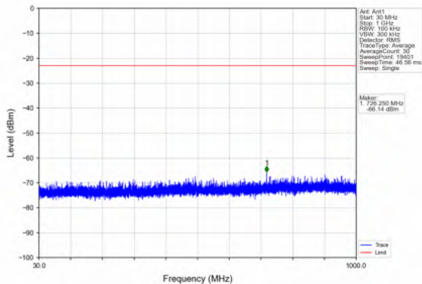
n41_30kHz_SISO_NTNV_20MHz_CP-OFDM QPSK_2679.99MHz_Inner_1RB_Right
