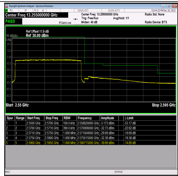
Band7_20MHz_16QAM_21350_100RB#0
