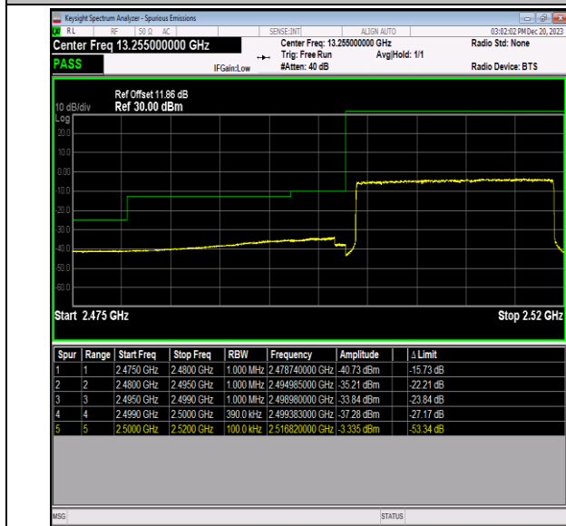
Band7_20MHz_16QAM_20850_100RB#0
