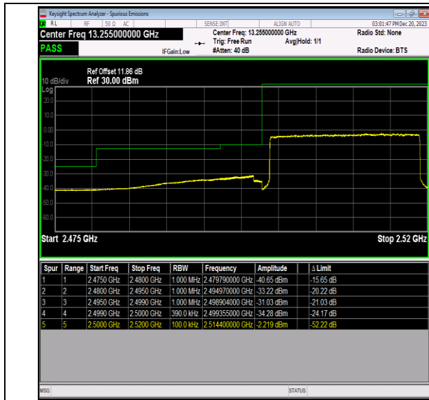
Band7_20MHz_QPSK_20850_100RB#0
