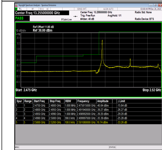
Band7_20MHz_64QAM_20850_1RB#0
