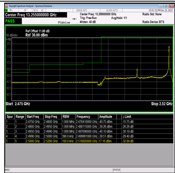
Band7_20MHz_64QAM_20850_1RB#99
