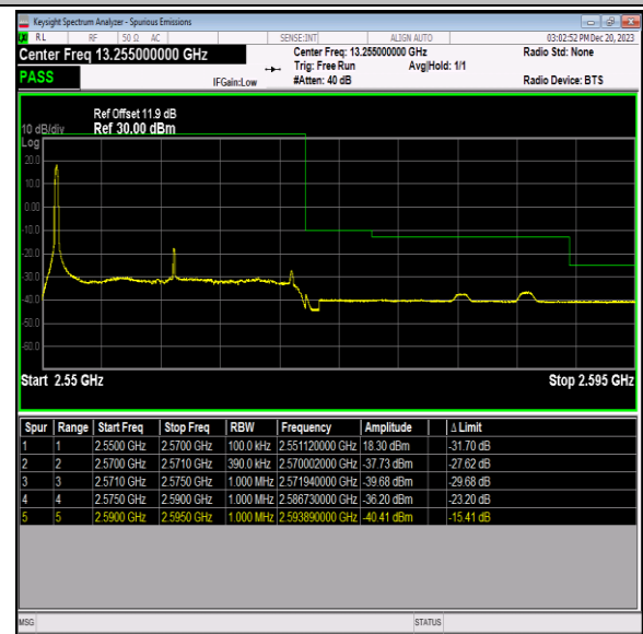
Band7_20MHz_16QAM_21350_1RB#0
