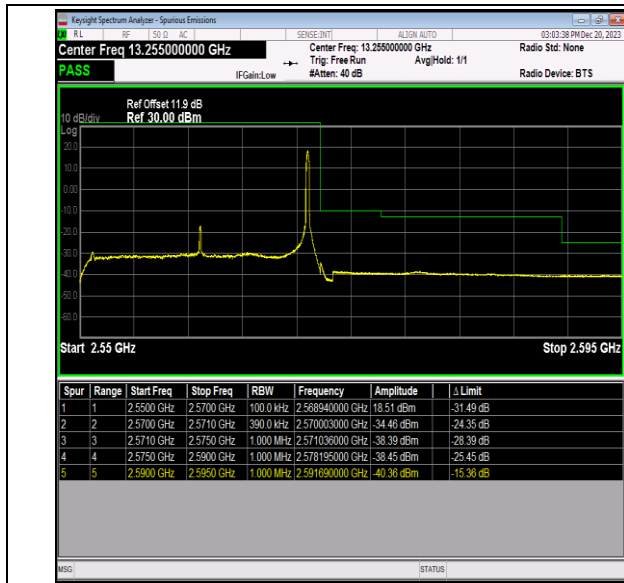
Band7_20MHz_16QAM_21350_1RB#99
