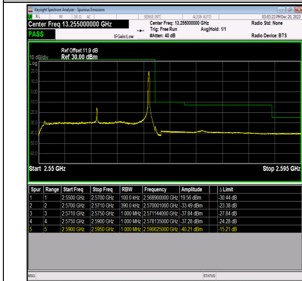
Band7_20MHz_QPSK_21350_1RB#99
