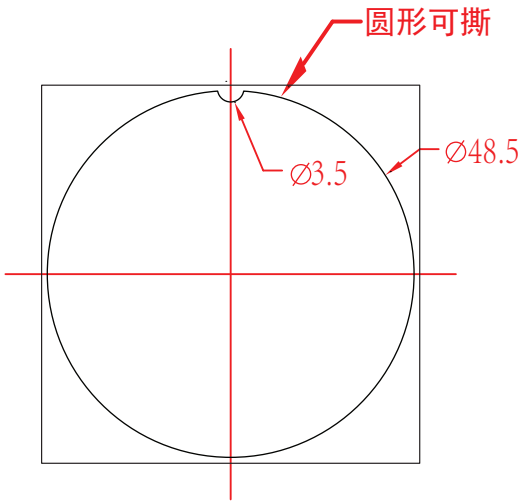
标贴尺寸图
