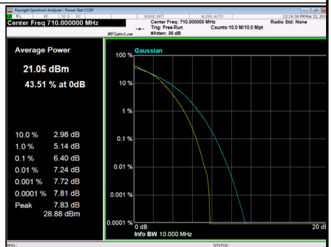
FDD17_10MHz_710_fullRB_Q16
