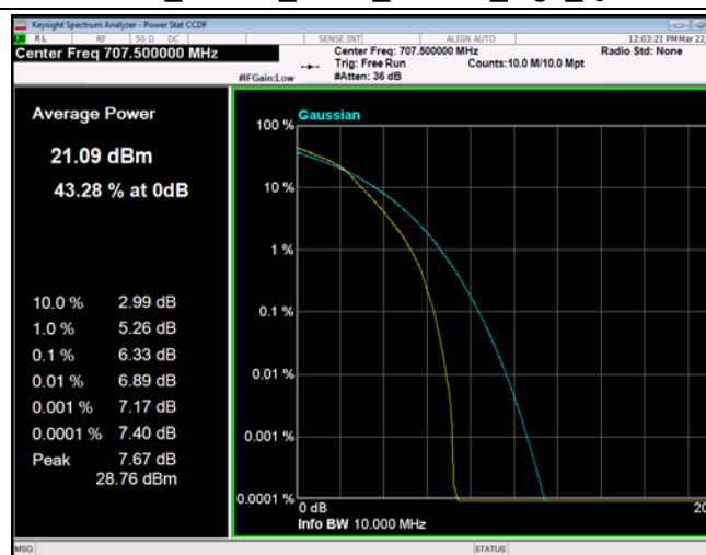
FDD12_10MHz_707.5_OneRB_high_Q16
