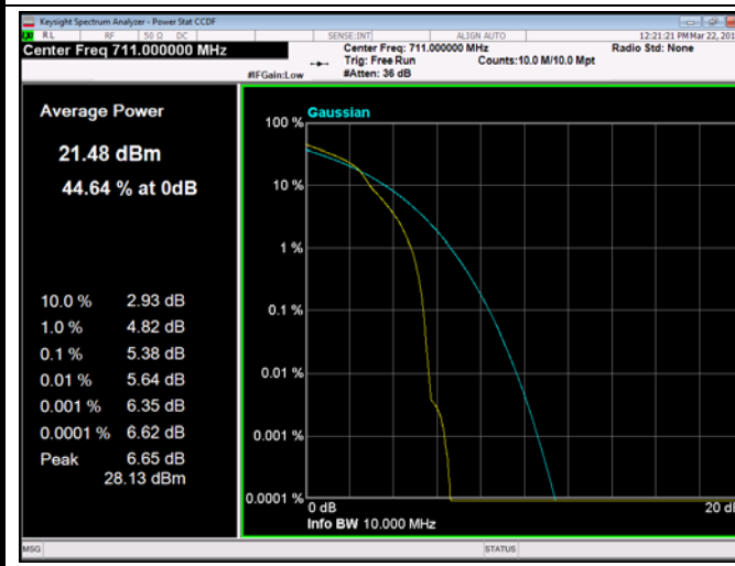
FDD17_10MHz_711_OneRB_high_Q16
