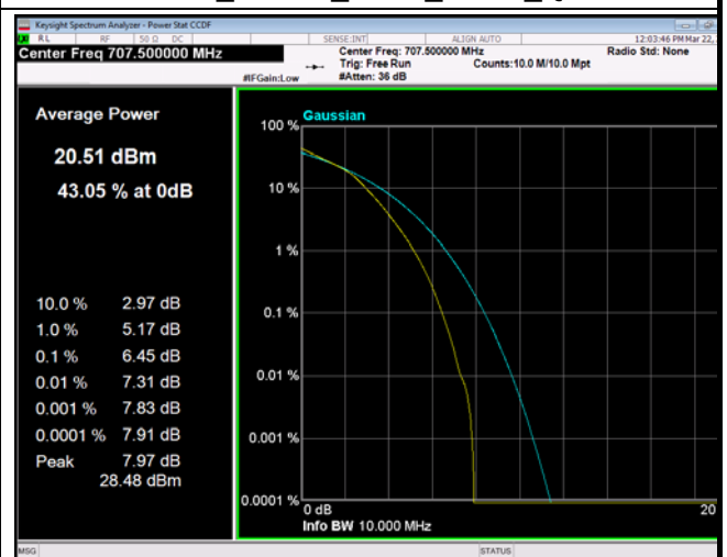
FDD12_10MHz_707.5_fullRB_Q16
