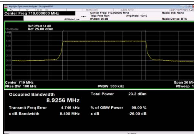
FDD17_MidRange_10MHz_710MHz_QPSK
