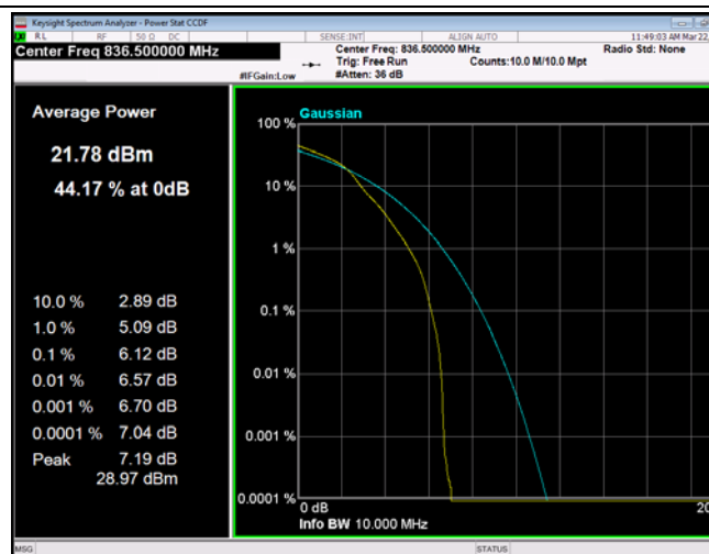
FDD05_10MHz_836.5_OneRB_high_Q16
