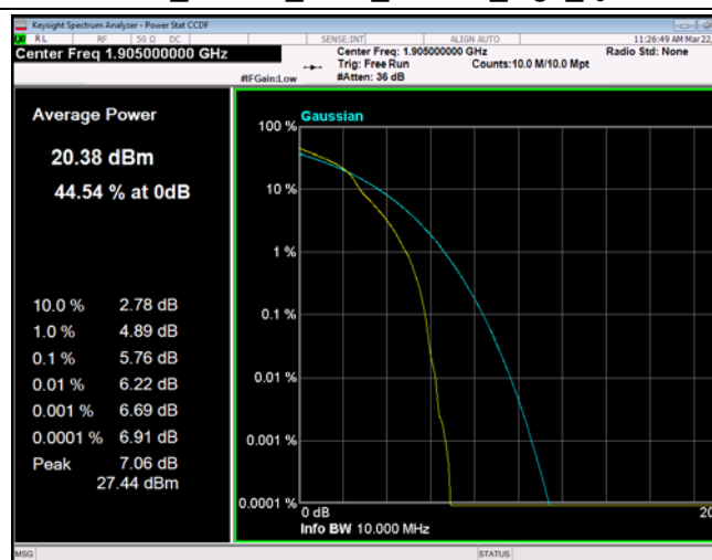
FDD02_10MHz_1905_OneRB_high_Q16
