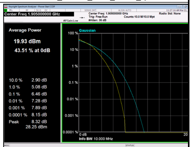
FDD02_10MHz_1905_fullRB_Q16
