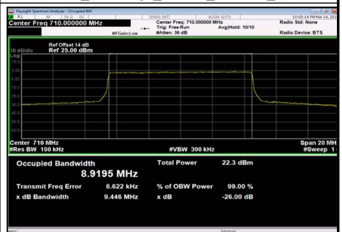
FDD17_MidRange_10MHz_710MHz_Q16
