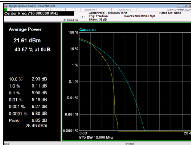
FDD17_10MHz_710_OneRB_high_Q16
