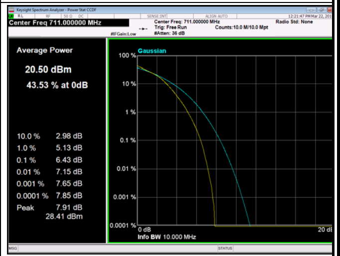
FDD17_10MHz_711_fullRB_Q16
