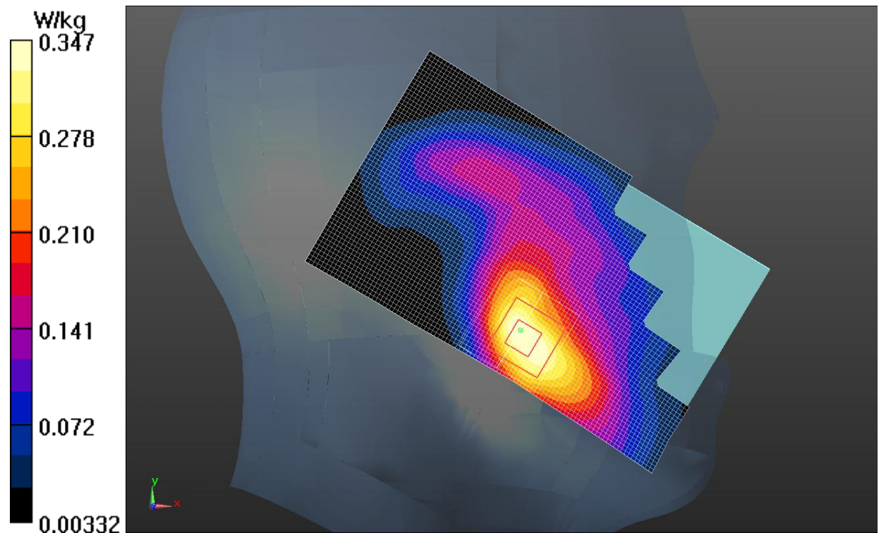
Fig.7 WCDMA1900 CH9262
