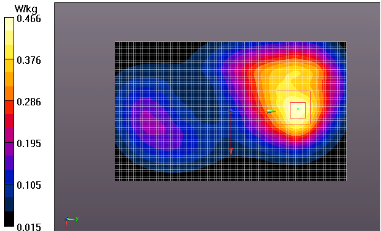
Fig.8 WCDMA1900 CH9262
