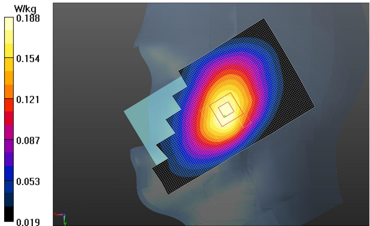
Fig.5 WCDMA 850 CH4182
