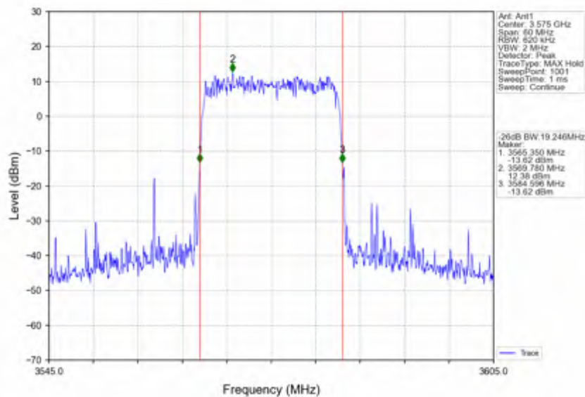
Band42c_20MHz_QPSK_MCH_3575MHz_RB_100_0_NTNV
