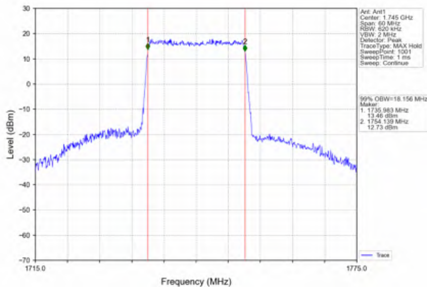
Band66_20MHz_QPSK_MCH_1745MHz_RB_100_0_NTNV
