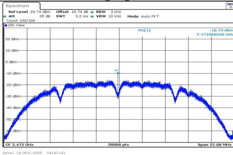
11B_Ant1_2472
