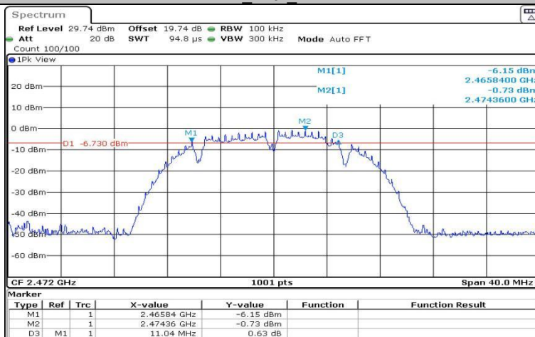
11B_Ant1_2472
