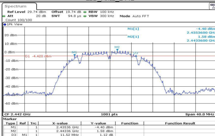
11B_Ant1_2442
