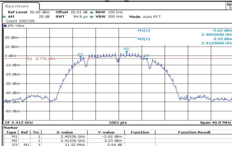
11B_Ant1_2412
