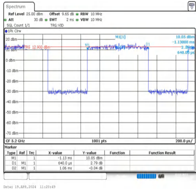
NTNV-11AX20MIMO-Ant2-5200
