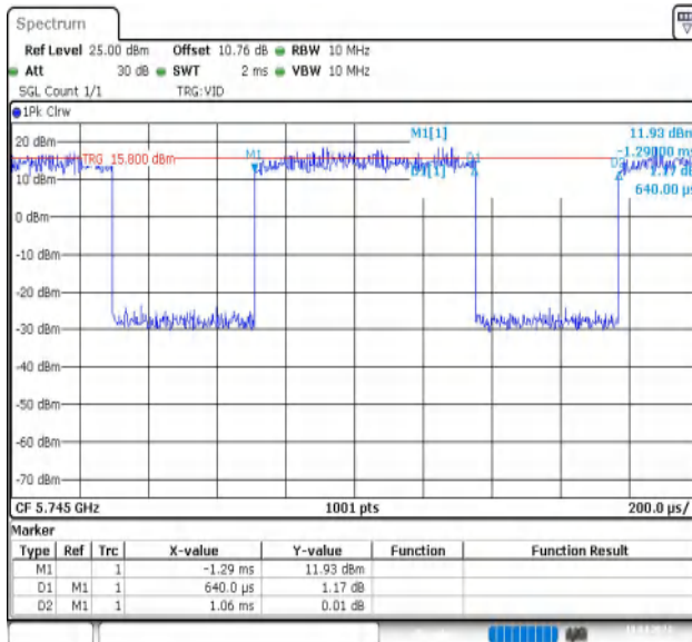
NTNV-11AX20MIMO-Ant1-5745
