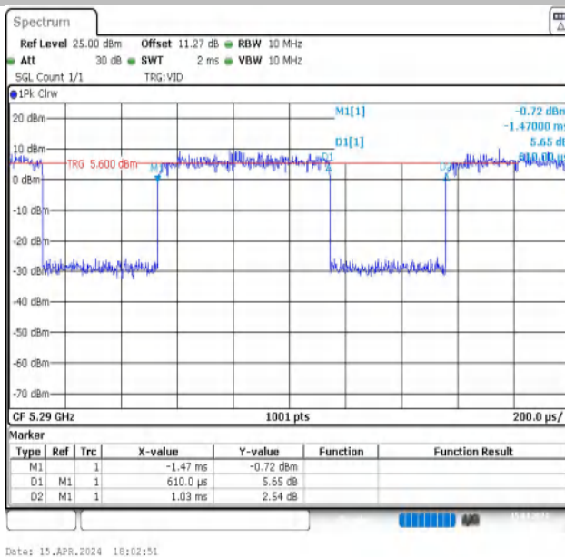
NTNV-11AX80MIMO-Ant1-5290
