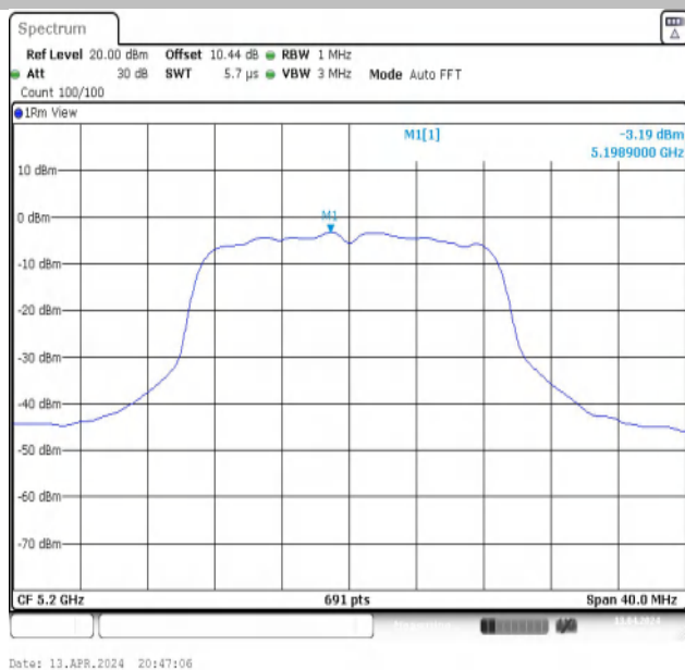
11N20MIMO-Ant1-5200-PASS
