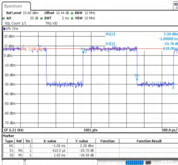
NTNV-11AX80MIMO-Ant1-5210
