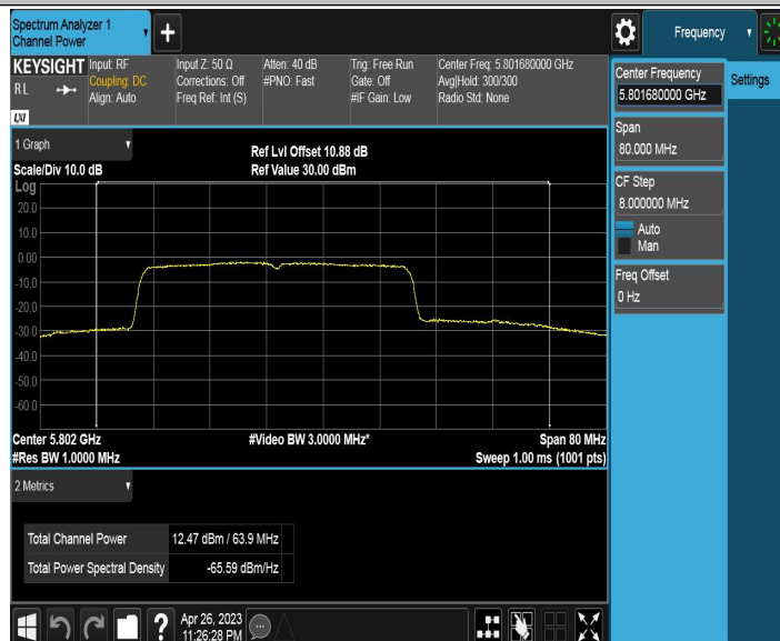
11AX40ISO_Ant2_5795
