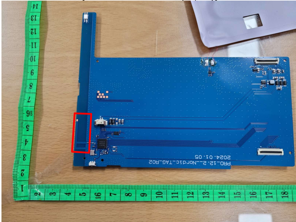
{NFC Antenna(RX)}
