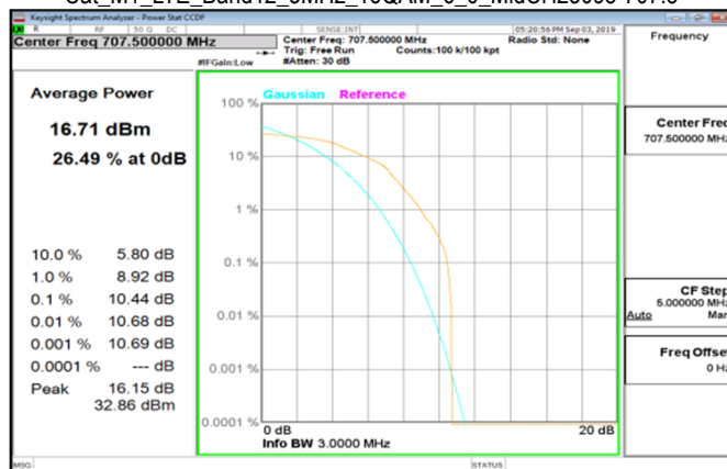
Cat M1 LTE_Band12_3MHz_16QAM_6_0_MidCH23095-707.5
