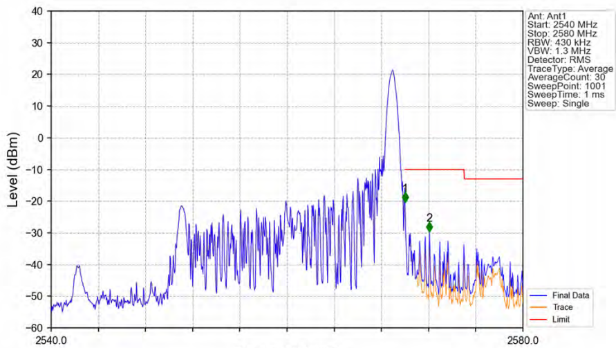
Band7_20MHz_QPSK_HCH_2560MHz_RB_1_99_NTNV
