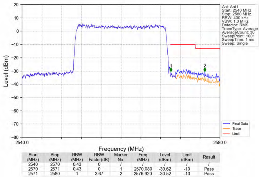
Band7_20MHz_16QAM_HCH_2560MHz_RB_100_0_NTNV
