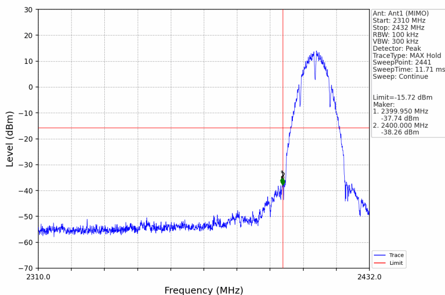
802.11b_LCH_2412MHz_Ant1 (MIMO)_NTNV
