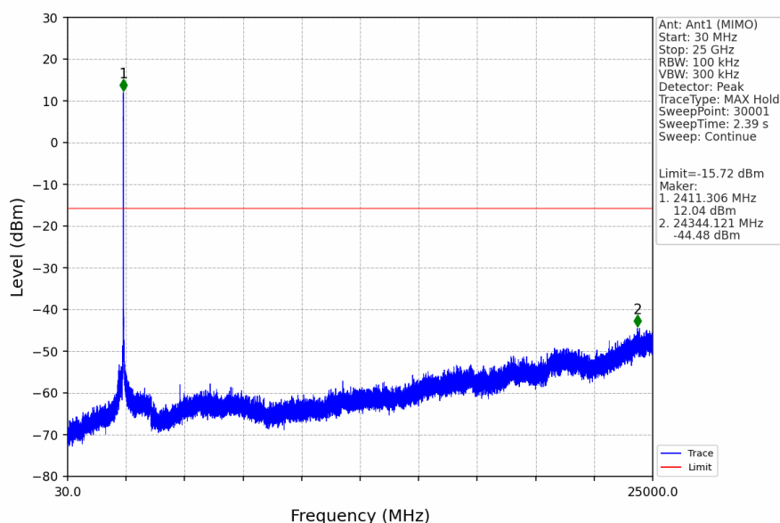
802.11b_LCH_2412MHz_Ant1 (MIMO)_NTNV
