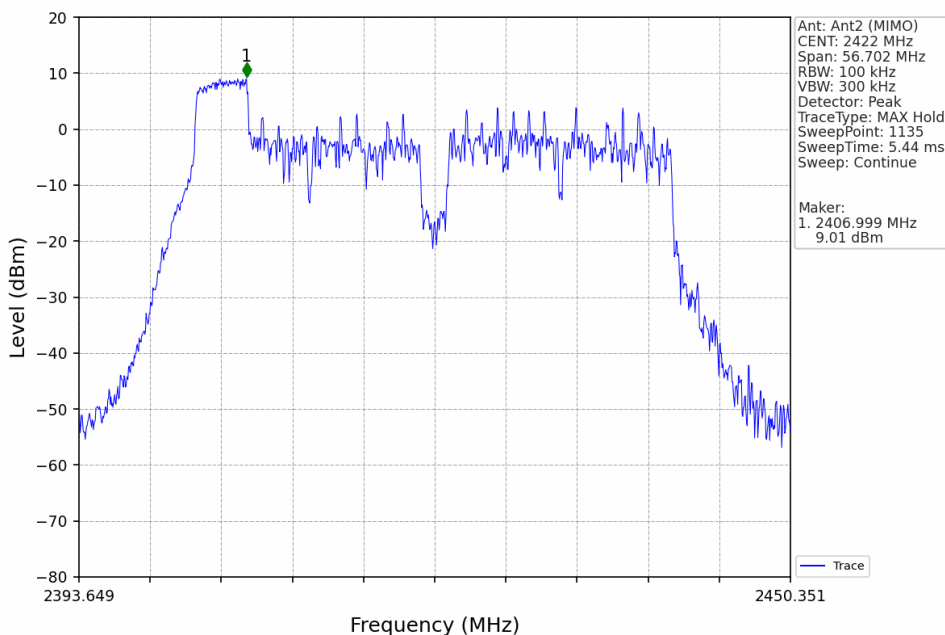
802.11ax(HEW40)_LCH_2422MHz_RU52_Left_Ant2 (MIMO)_NTNV
