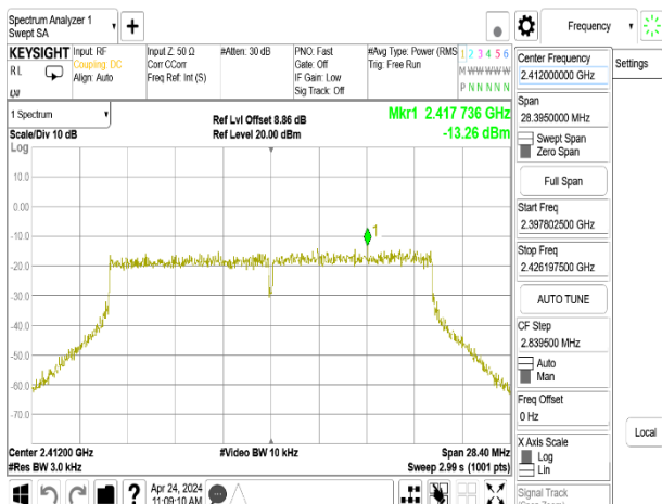
802.11be_20MHz_Chain0_2412MHz_106+26_MRUI
