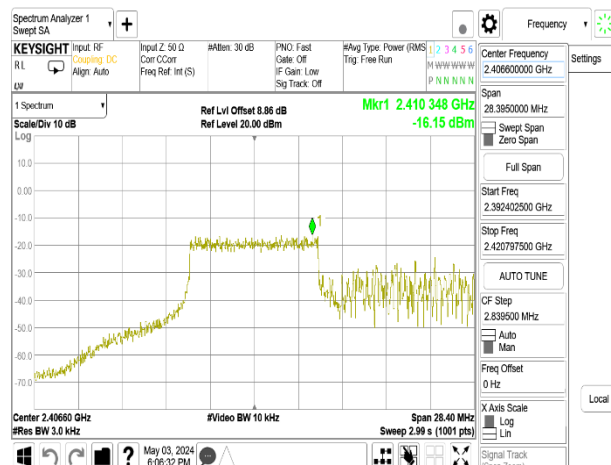
802.11be_20MHz_Chain0_2412MHz_RU26_0
