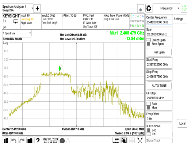
802.11be_20MHz_Chain0_2412MHz_52+26_MRUI
