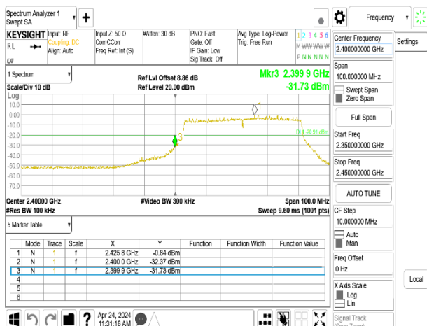
802.11be_40MHz_Chain1_2422MHz
