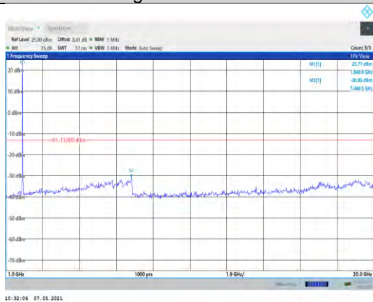
Band2-3MHz-QPSK-18615-1RB#0- Range2:1000~20000MHz
