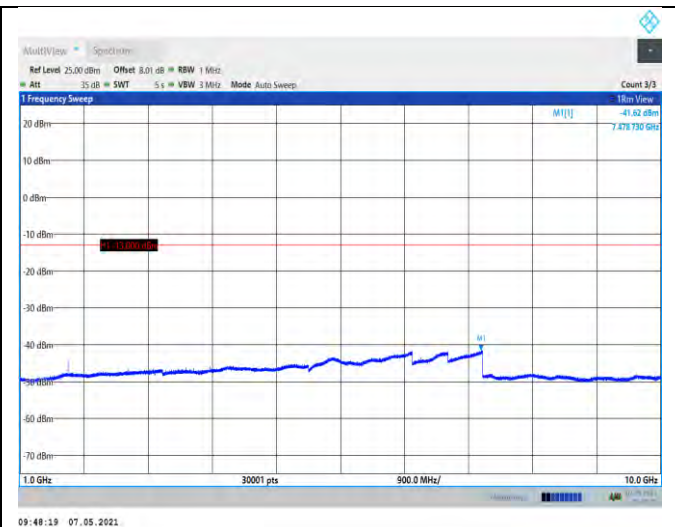
EGPRS850-128-1000~10000MHz
