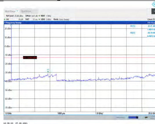
Band2-5MHz-QPSK-19175-1RB#0- Range2:1000~20000MHz
