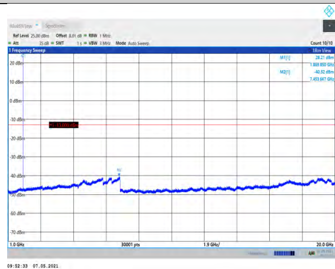
GSM1900-661-1000~20000MHz
