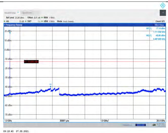
Band4-1312-1000~20000MHz
