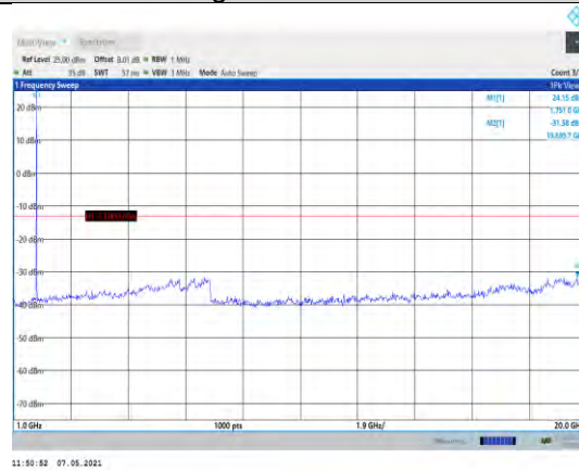
Band4-1.4MHz-QPSK-20393-1RB#0- Range2:1000~20000MHz
