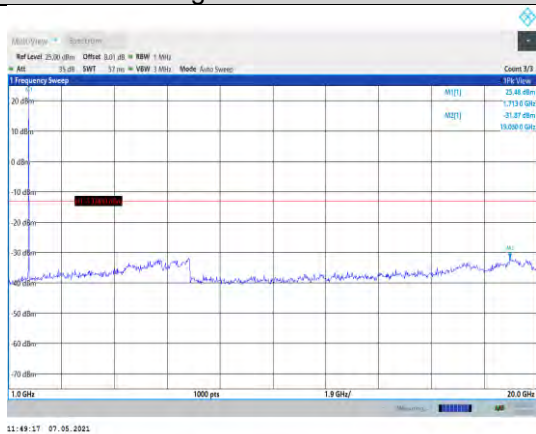
Band4-1.4MHz-QPSK-19957-1RB#0- Range2:1000~20000MHz
