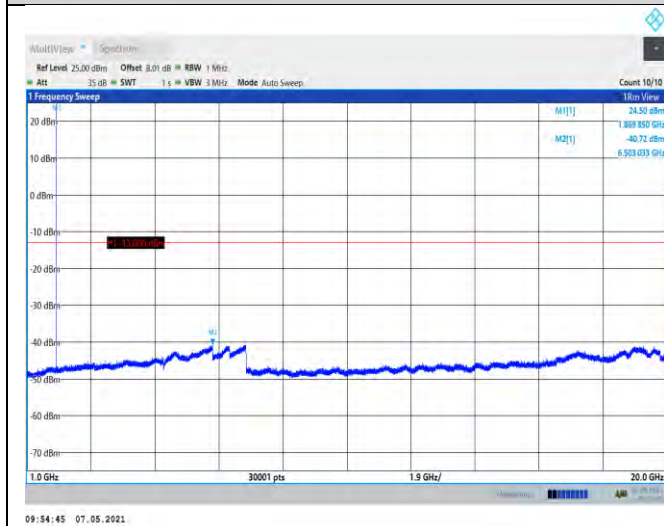
EGPRS1900-810-1000~20000MHz
