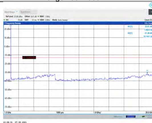
Band2-15MHz-QPSK-19125-1RB#0- Range2:1000~20000MHz
