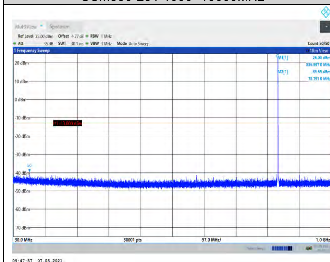
EGPRS850-128-30~1000MHz
