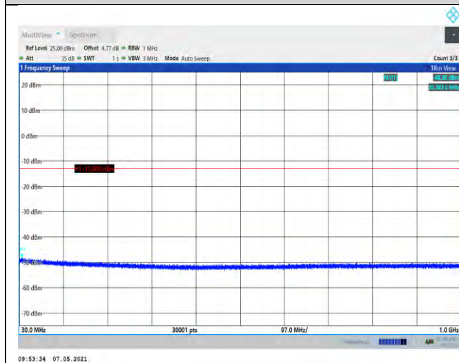
EGPRS1900-512-30~1000MHz
