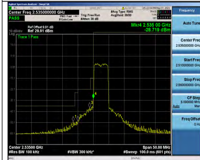
Band41-5MHz-QPSK-40065-25RB#0
