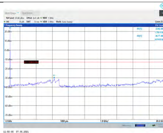
Band4-1.4MHz-QPSK-20175-1RB#0- Range2:1000~20000MHz
