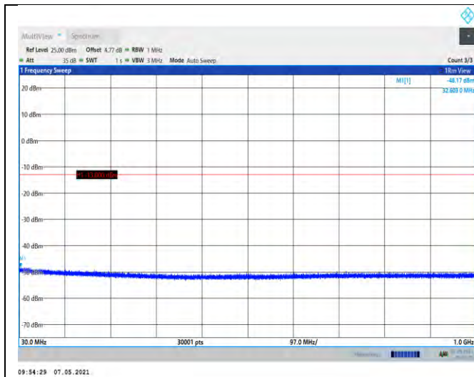
EGPRS1900-810-30~1000MHz
