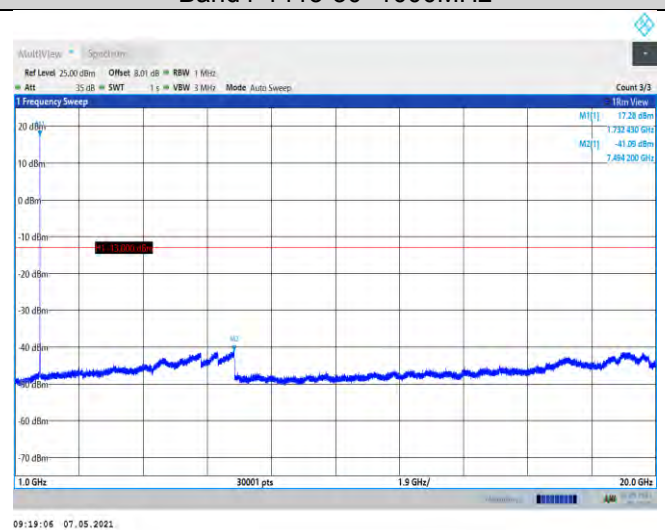
Band4-1413-1000~20000MHz
