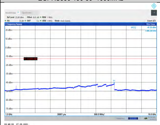
EGPRS850-190-1000~10000MHz
