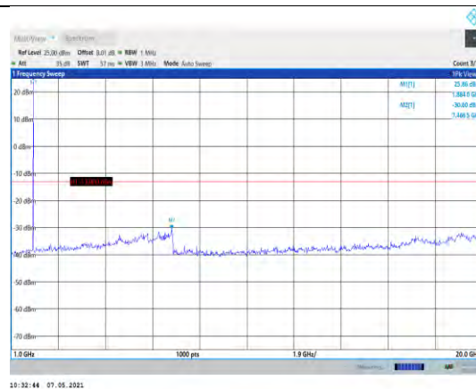
Band2-3MHz-QPSK-18900-1RB#0- Range2:1000~20000MHz
