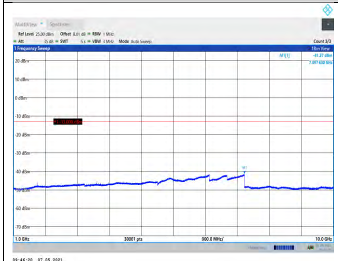
GSM850-128-1000~10000MHz
