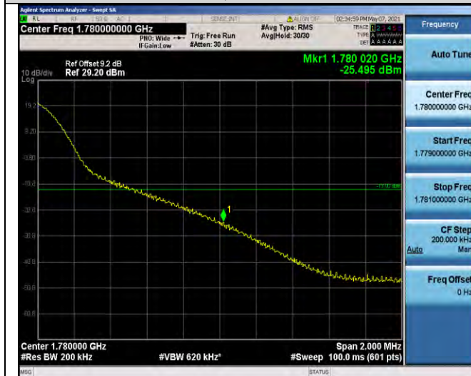
Band66-20MHz-QPSK-132572-1RB#99
