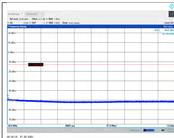
Band4-1513-30~1000MHz
