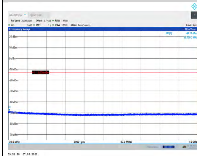
GSM1900-512-30~1000MHz
