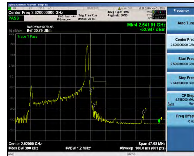
Band38-20MHz-QPSK-38150-1RB#99
