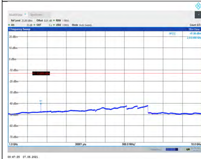
GSM850-251-1000~10000MHz
