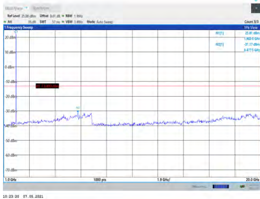
Band2-1.4MHz-QPSK-19193-1RB#0- Range2:1000~20000MHz
