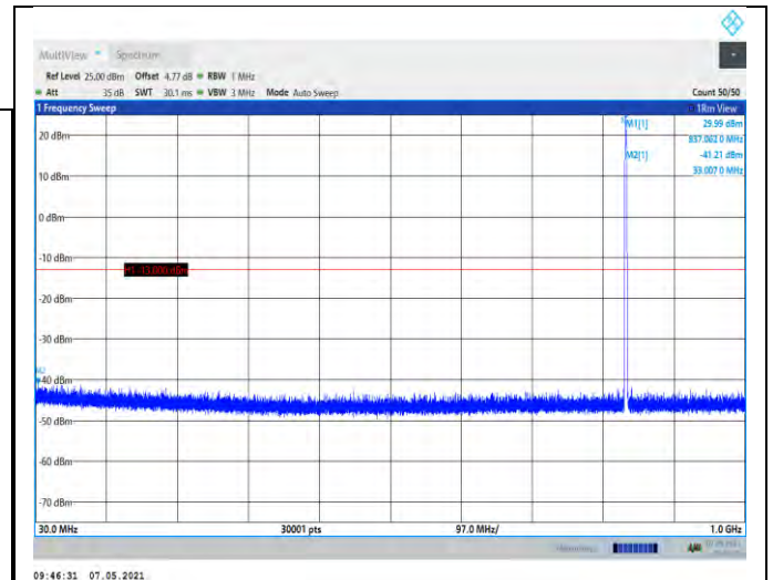
GSM850-190-30~1000MHz
