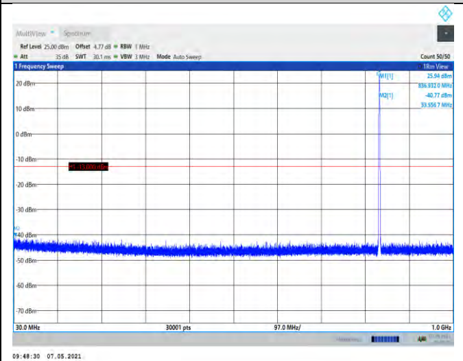
EGPRS850-190-30~1000MHz
