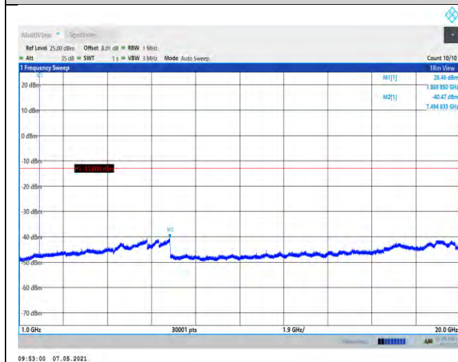
GSM1900-810-1000~20000MHz
