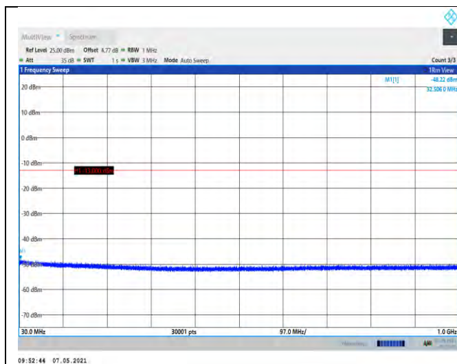
GSM1900-810-30~1000MHz
