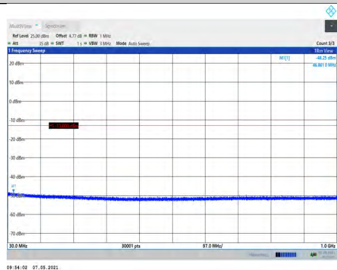
EGPRS1900-661-30~1000MHz
