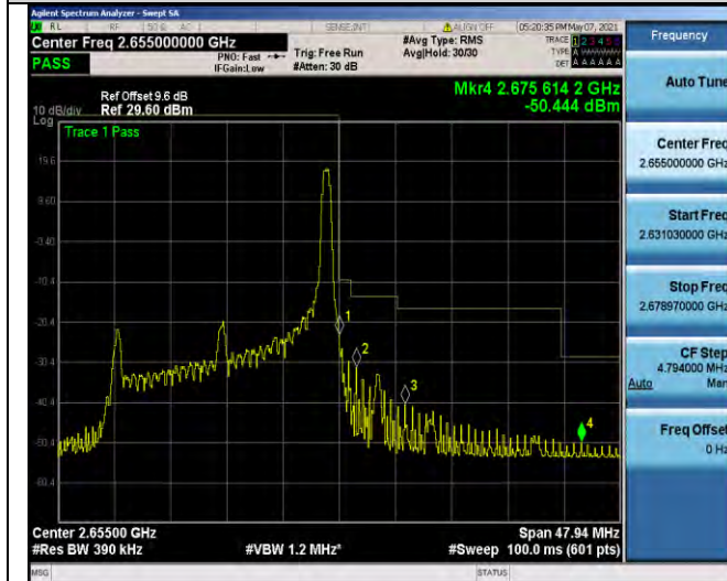
Band41-20MHz-QPSK-41140-1RB#99
