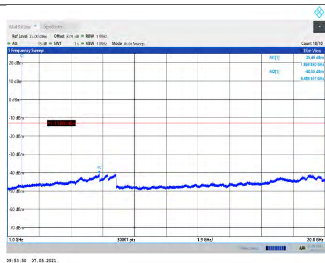
EGPRS1900-512-1000~20000MHz
