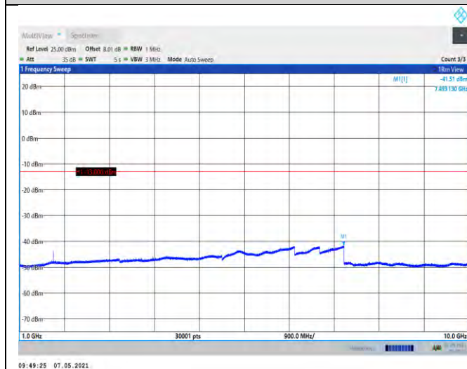
EGPRS850-251-1000~10000MHz
