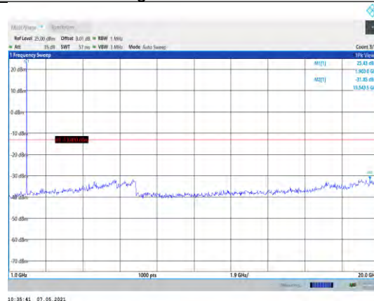
Band2-5MHz-16QAM-19175-1RB#0- Range2:1000~20000MHz
