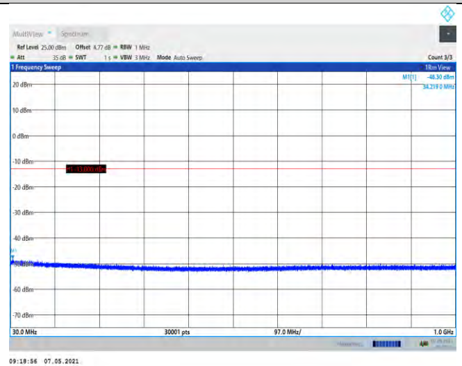
Band4-1413-30~1000MHz
