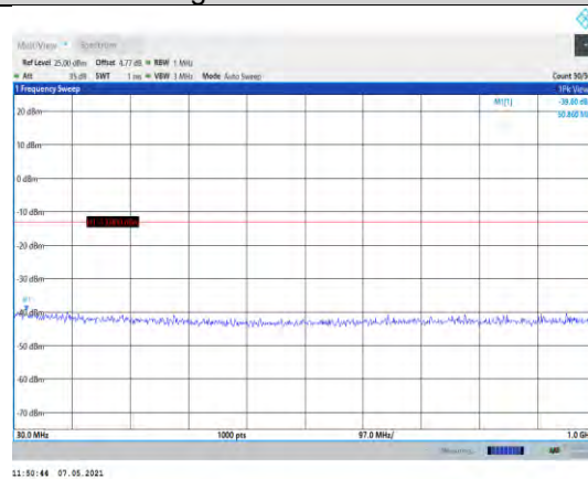
Band4-1.4MHz-QPSK-20393-1RB#0- Range1:30~1000MHz
