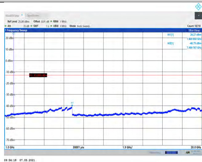
EGPRS1900-661-1000~20000MHz
