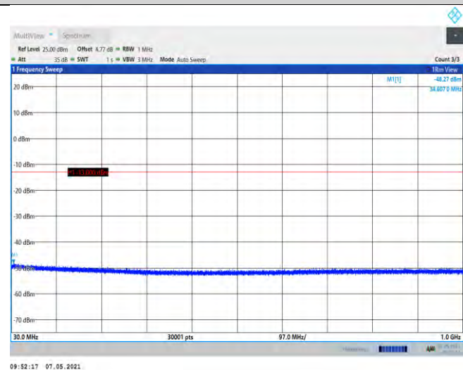
GSM1900-661-30~1000MHz
