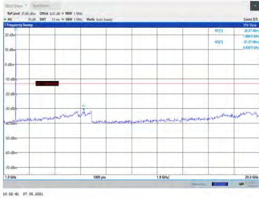
Band2-1.4MHz-QPSK-18900-1RB#0- Range2:1000~20000MHz
