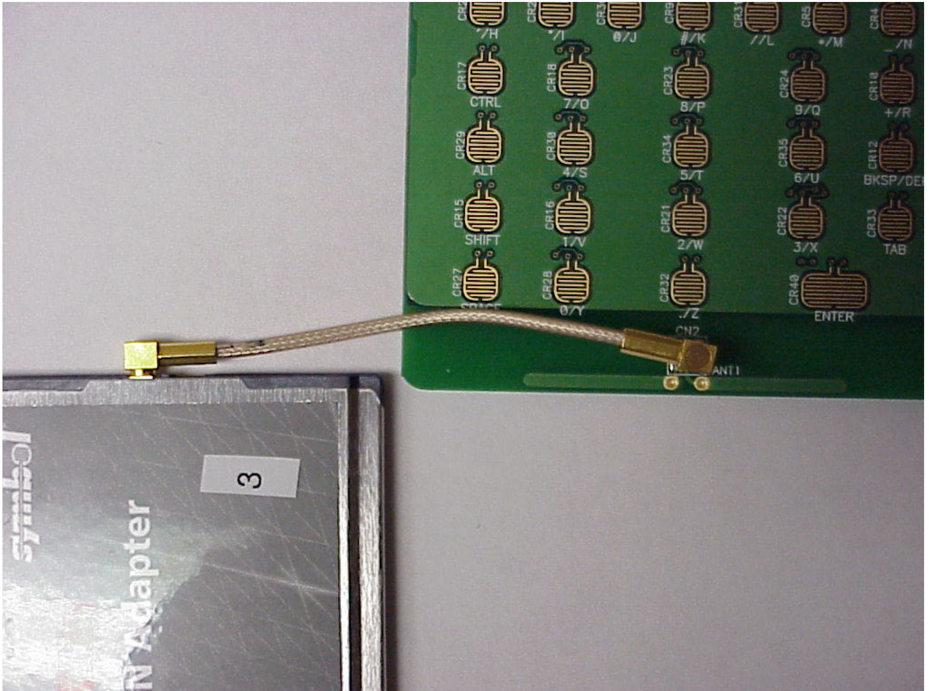
Antenna
