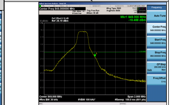
Band5-3MHz-QPSK-20635-1RB#14
