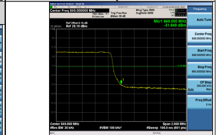
Band5-3MHz-QPSK-20635-15RB#0
