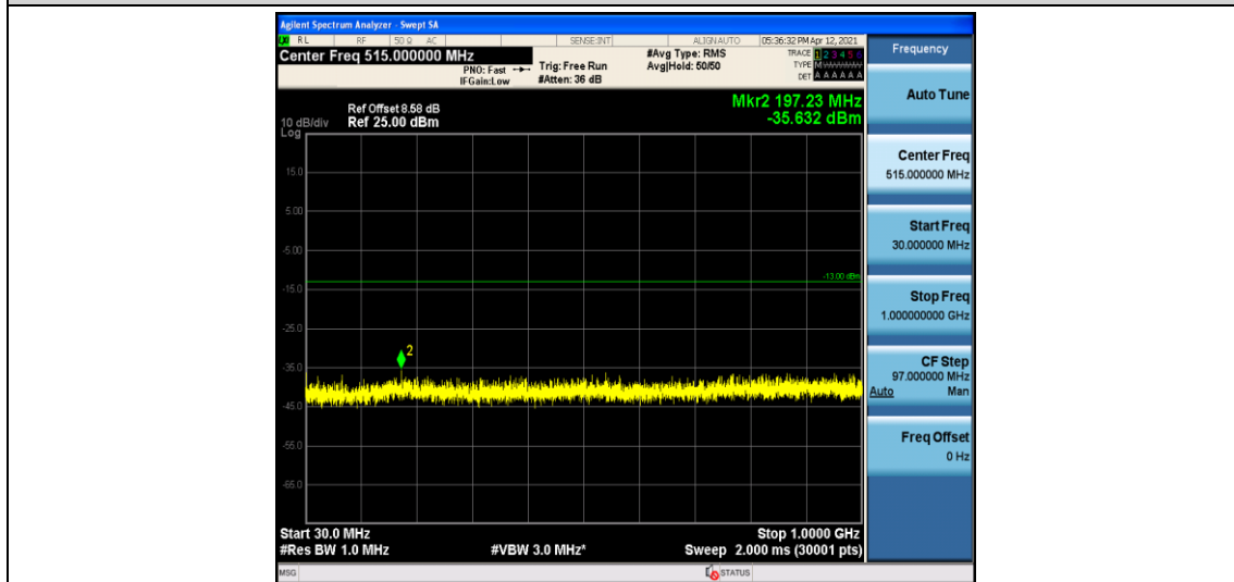
Band5-5MHz-QPSK-20525-1-0-Low-30-1000--35.63-PASS
