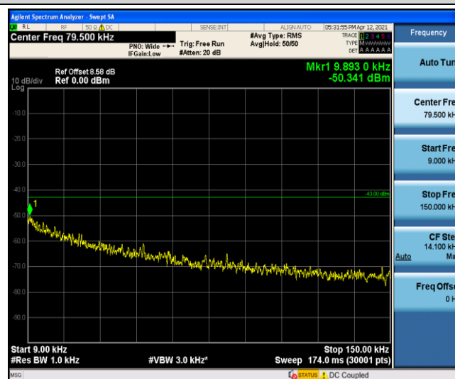
Band5-5MHz-QPSK-20425-1-0-Low-0.009-0.15--50.34-PASS
