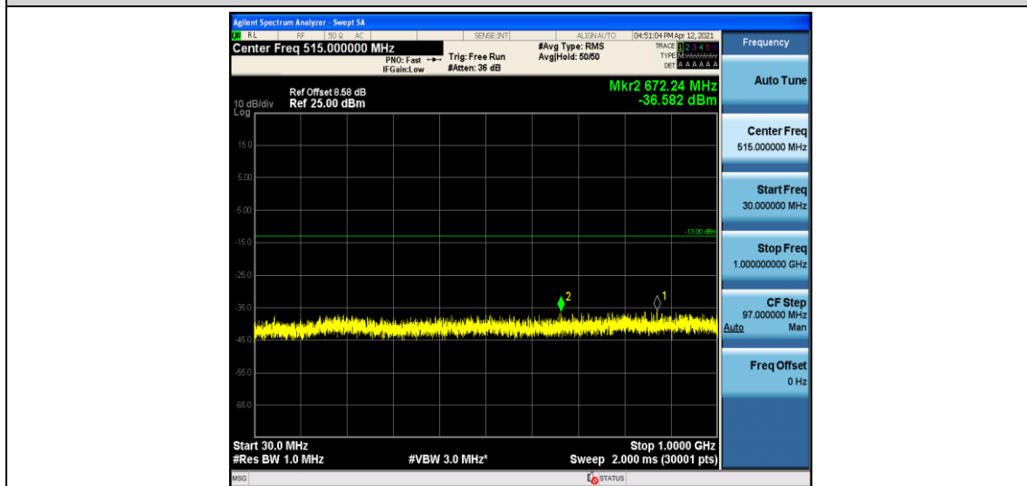
Band5-3MHz-QPSK-20525-1-0-Low-30-1000--36.58-PASS
