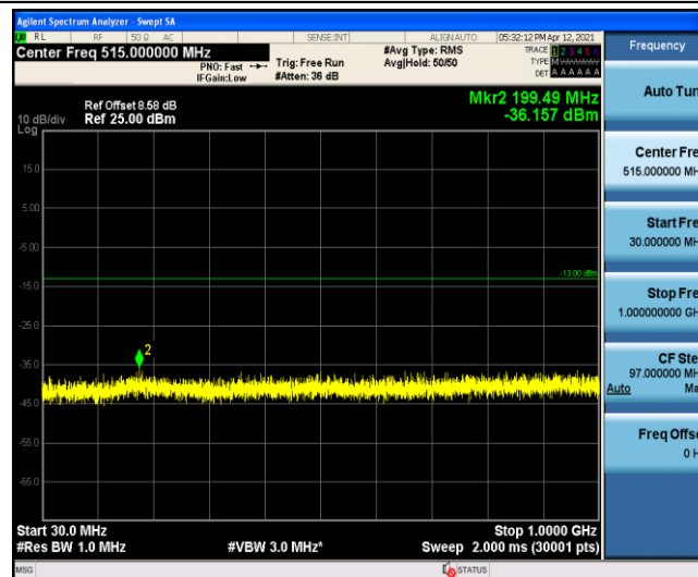
Band5-5MHz-QPSK-20425-1-0-Low-30-1000--36.16-PASS
