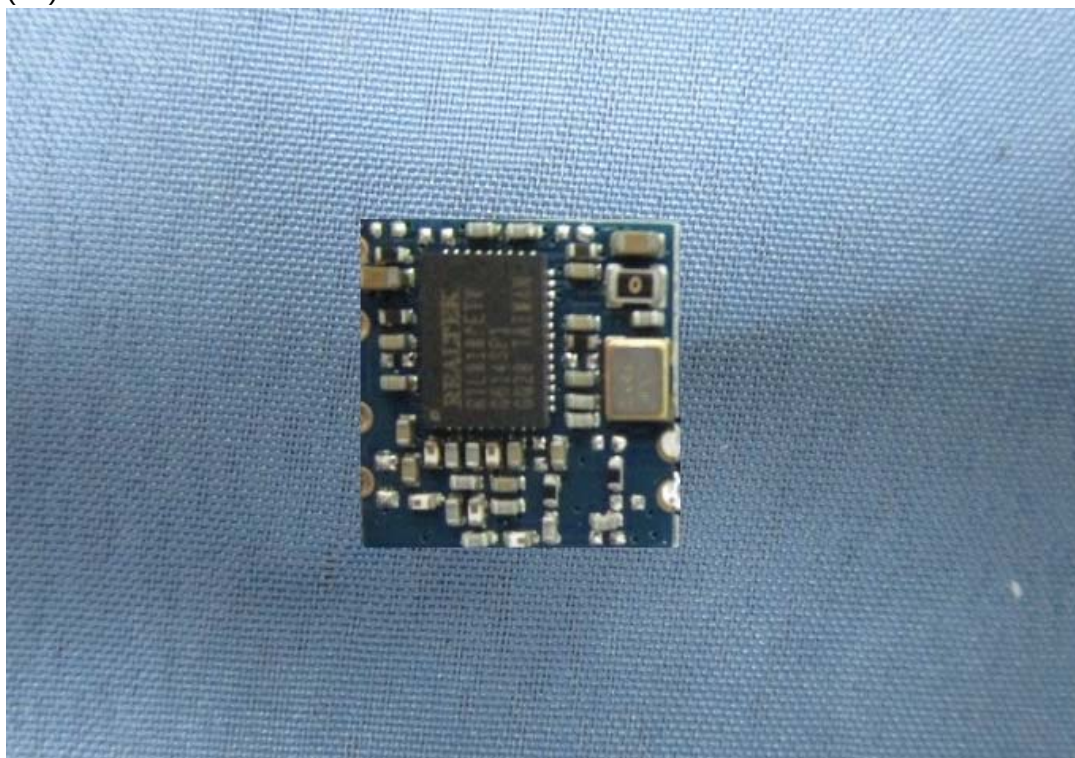
(13) EUT Photo
