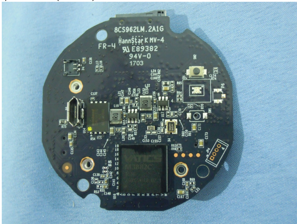
(10) EUT Photo (WiFi-MB)
