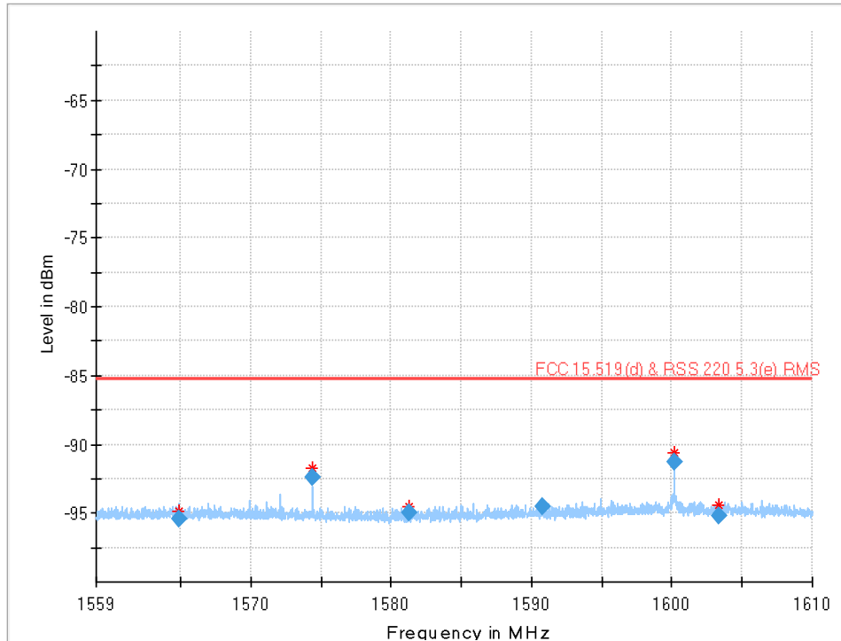
Plot 13: 1559 MHz to 1610 MHz (§15.519 (d), RSS-220 5.3.1(e)), UWB test mode
