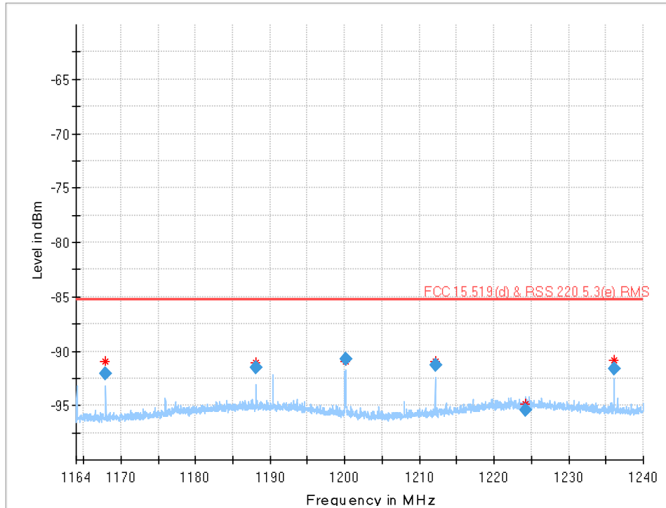
Plot 12: 1164 MHz to 1240 MHz (§15.519 (d), RSS-220 5.3.1(e)), UWB test mode
