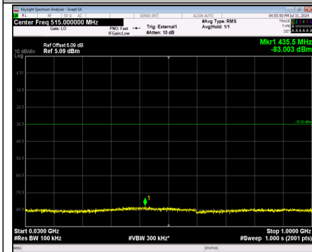
41-41-20MHz-20MHz-64QAM-64QAM-40641-40839-1R B#0-ORB#0-30~1000MHz-PASS
