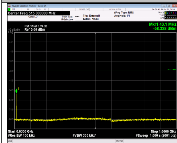
41-41-20MHz-20MHz-64QAM-64QAM-40641-40839-1R B#99-0RB#0-30~1000MHz-PASS
