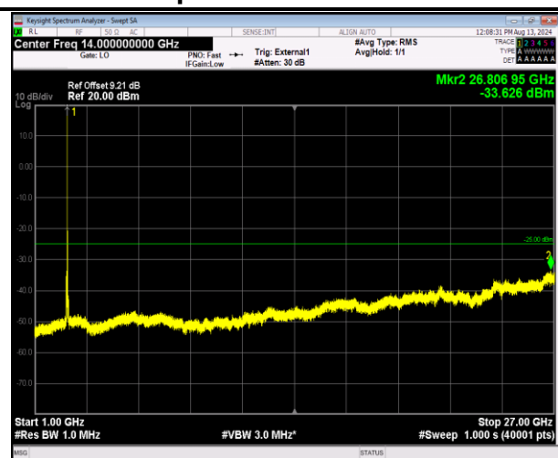
41-41-20MHz-20MHz-QPSK-QPSK-40942-41140-1RB#0- 0RB#0-1000~27000MHz-PASS
