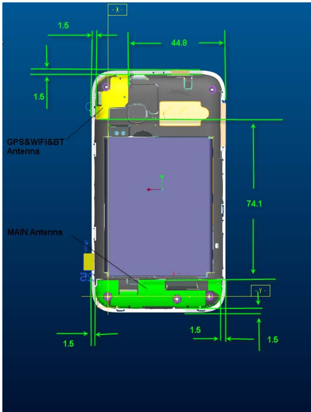
b: Antenna
