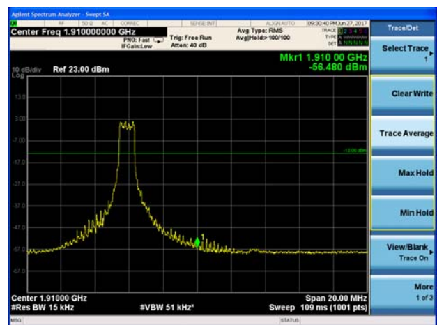
LTE Band 2 10MHz QPSK 1RB CH-High
