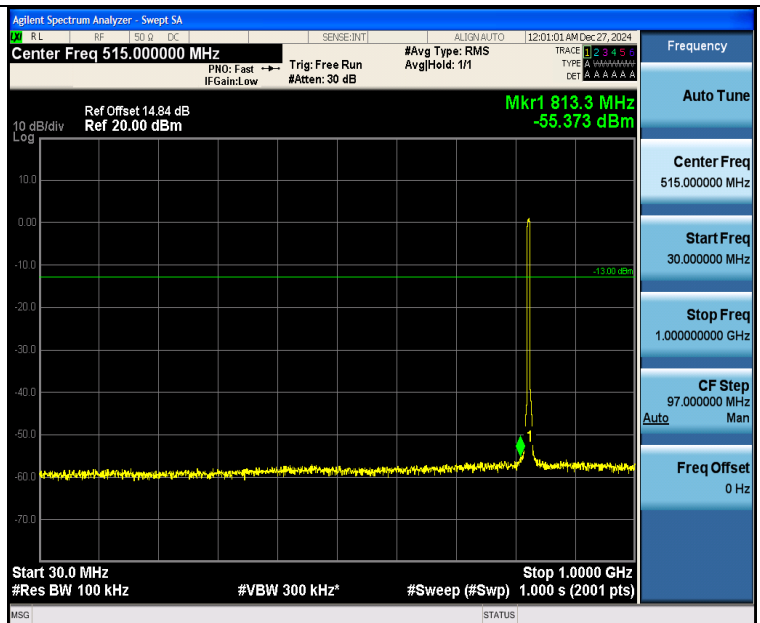
Band26 5MHz 16QAM 26815 25RB#0 30~1000 30~1000
