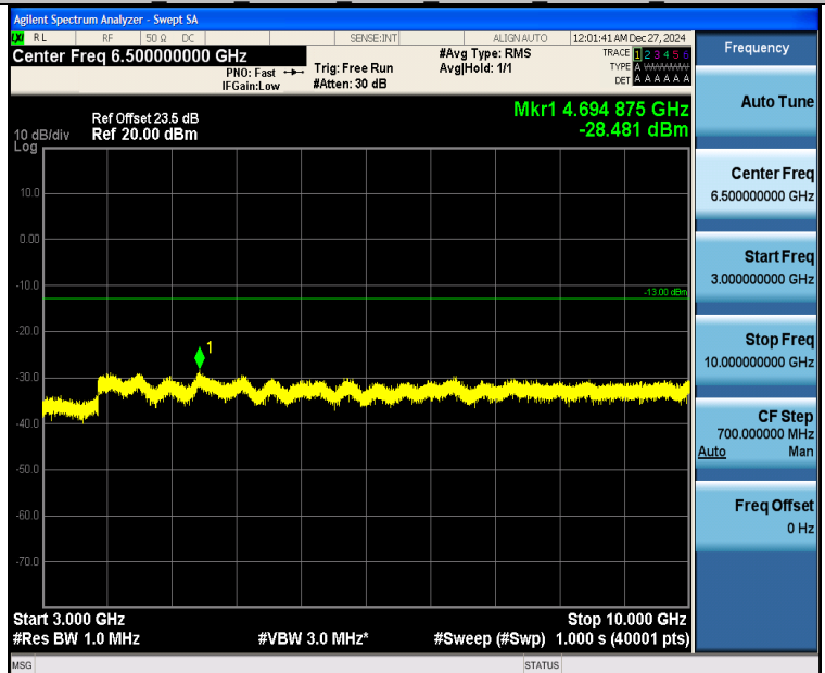
Band26 5MHz 16QAM 26815 25RB#0 3000~10000 3000~10000
