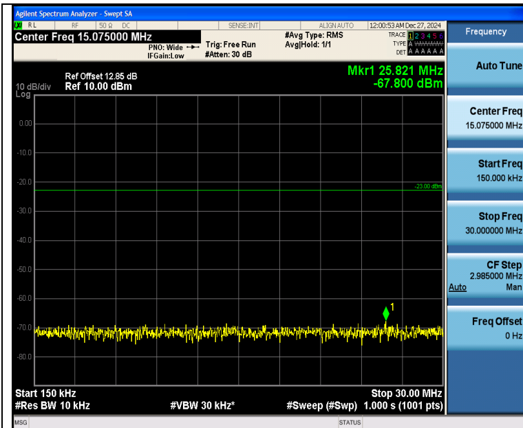
Band26 5MHz 16QAM 26815 25RB#0 0.15~30 0.15~30
