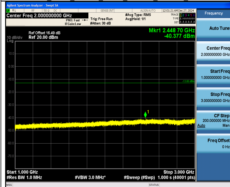
Band26 5MHz 16QAM 26815 25RB#0 1000~3000 1000~3000
