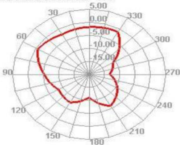
2500.000MHz E1
