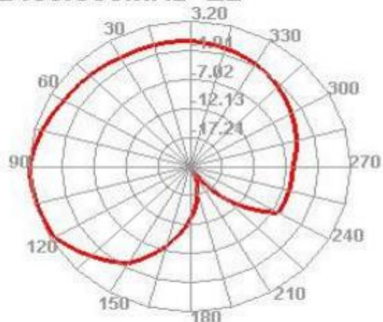
2400.000MHz E2
