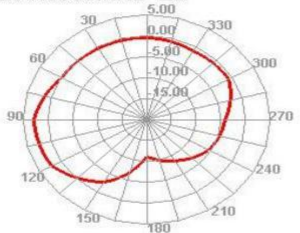
2500.000MHz E2
