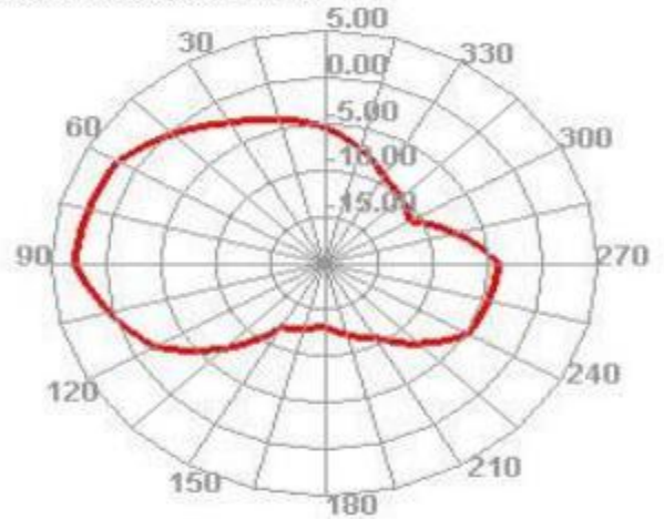
2500.000MHz H
