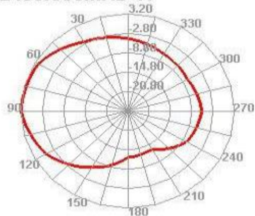
2400.000MHz H
