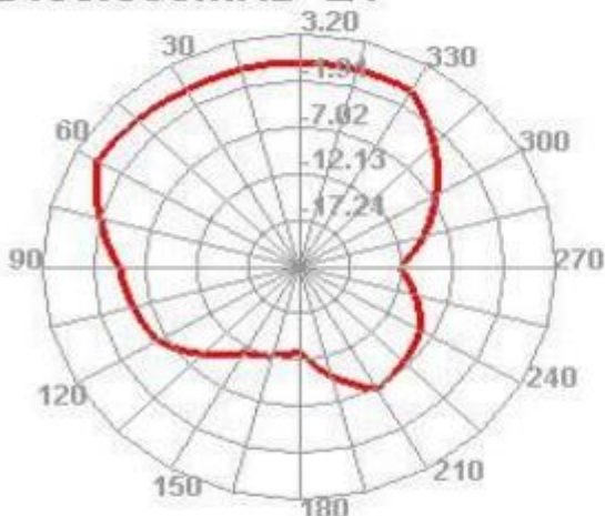
2400.000MHz E1
