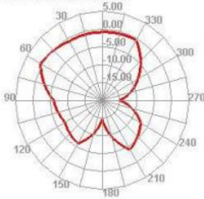
2450.000MHz E1
