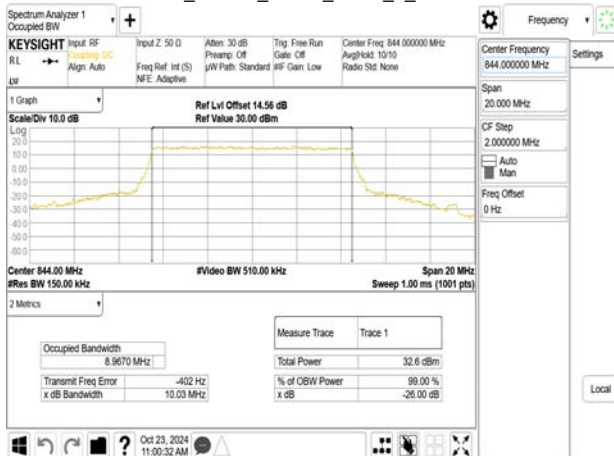
Band5_10MHz_QPSK_RB50_0_CH20600
