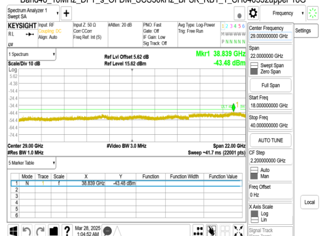
Band48_10MHz_DFT_s_OFDM_SCS30kHz_BPSK_RB1_1_CH646332upper 18G
