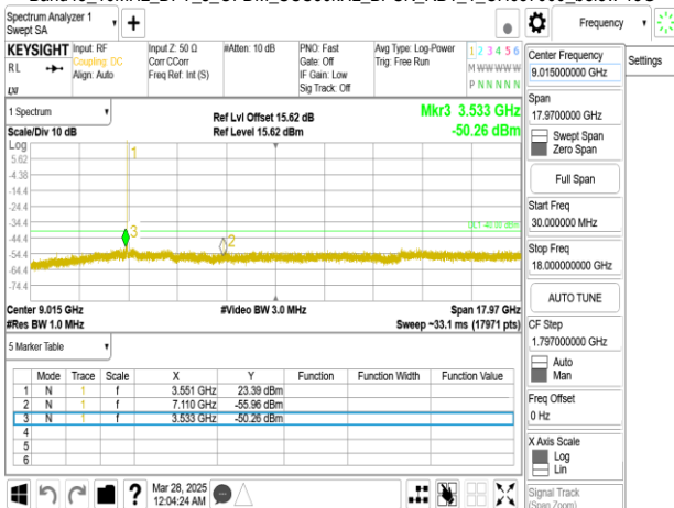
Band48_10MHz_DFT_s_OFDM_SCS30kHz_BPSK_RB1_1_CH637000upper 18G
