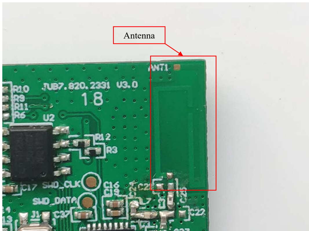
FIGURE 14 SMART PLUG (MODEL: CPLGSTDBLW1)(HVIN: CPLGSTDXCW1T) WLAN ANT
