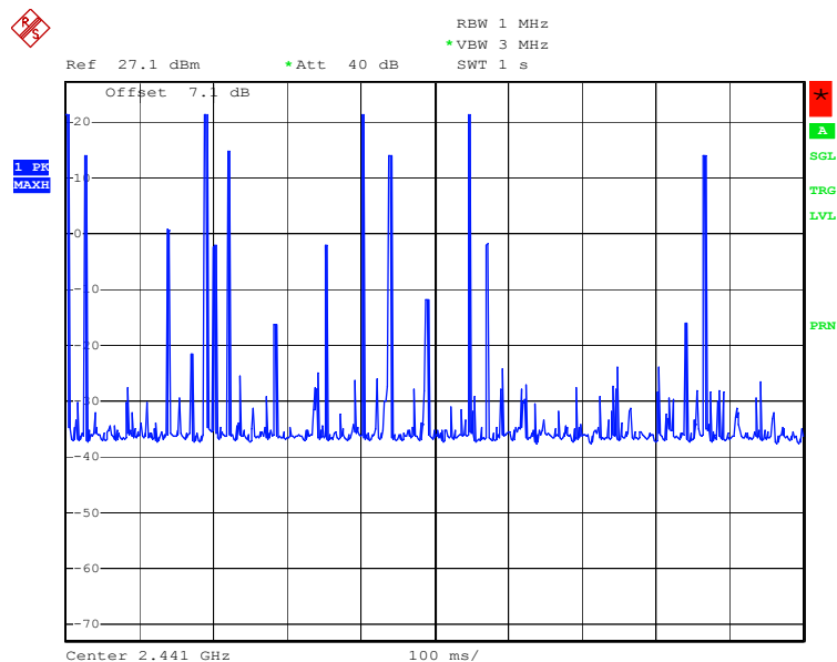
Figure 10. 4 DH 5 bursts
