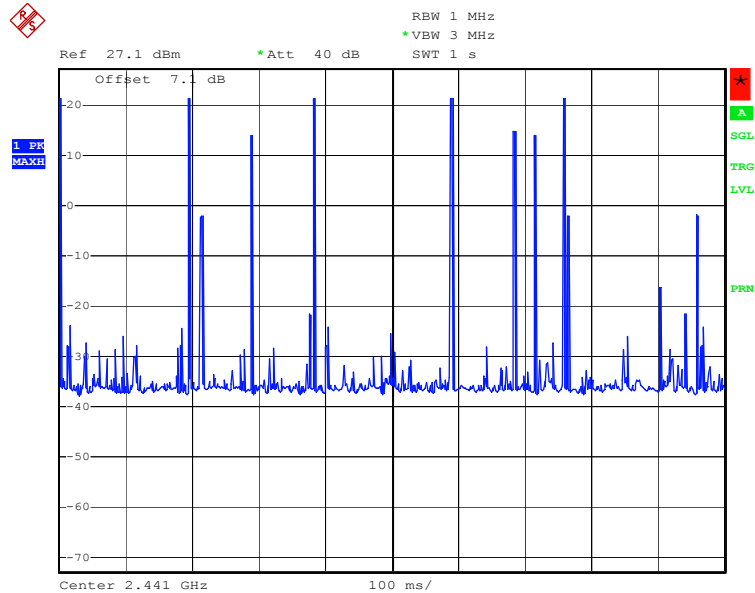
Figure 10. 4 DH 5 bursts
