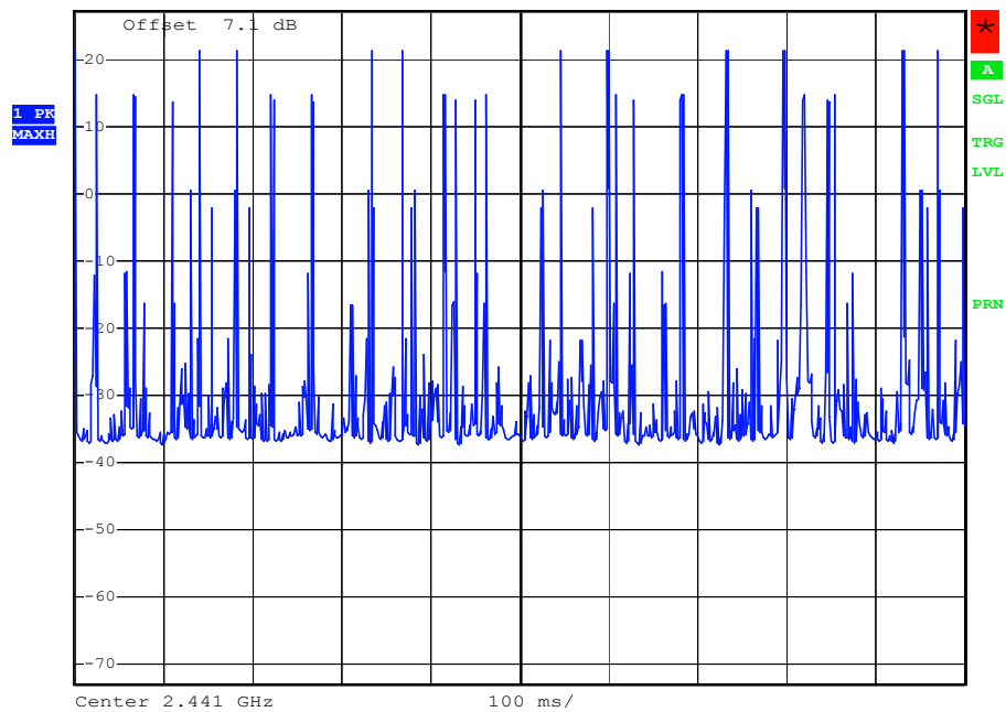
Figure 6. 10 DH 1 bursts
