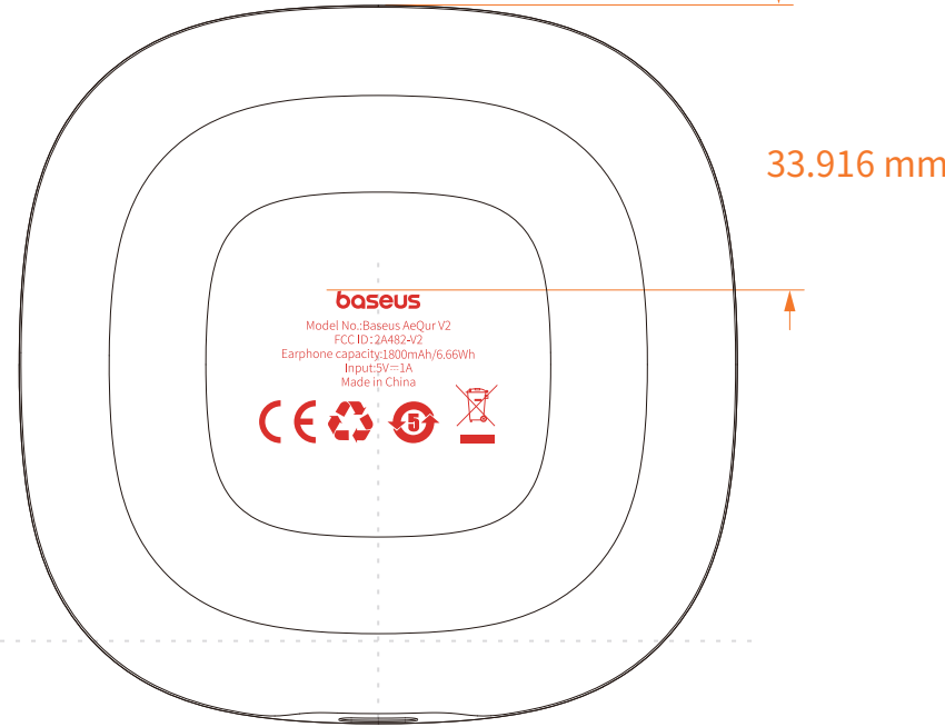
低视图
