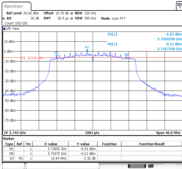
11AX20MIMO-Ant1-5745-PASS
