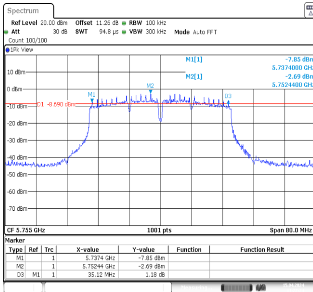
11N40MIMO-Ant1-5755-PASS
