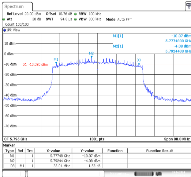
11AX40MIMO-Ant1-5795-PASS
