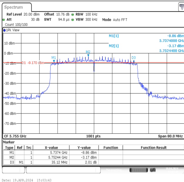
11AX40MIMO-Ant1-5755-PASS
