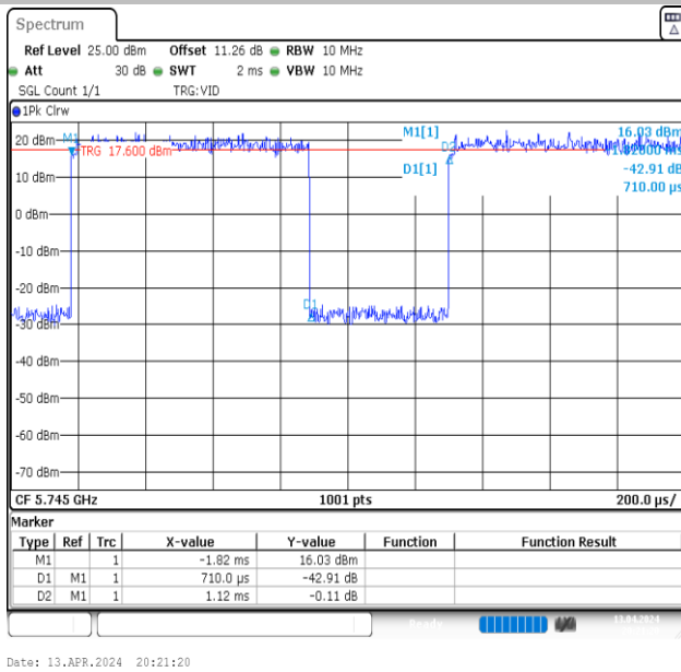
NTNV-11A-Ant1-5745
