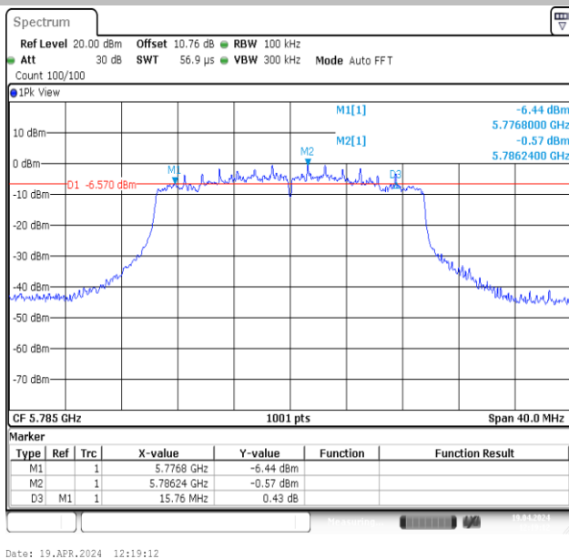
11AX20MIMO-Ant1-5785-PASS
