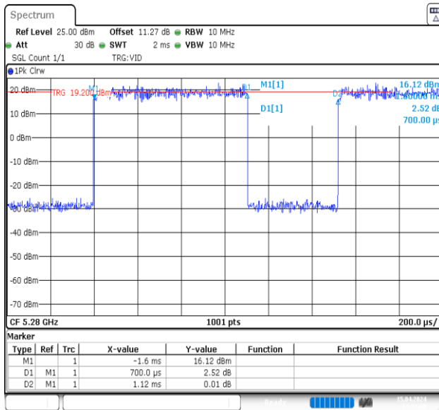
NTNV-11A-Ant1-5280
