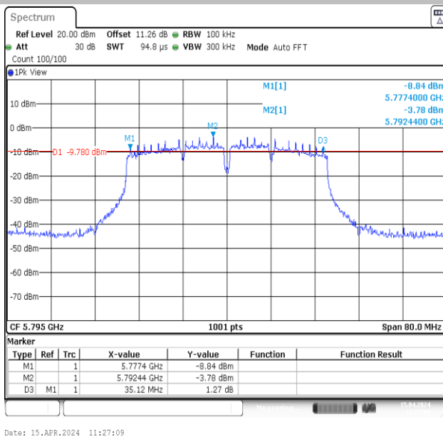
11N40MIMO-Ant1-5795-PASS
