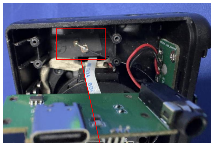
antenna
