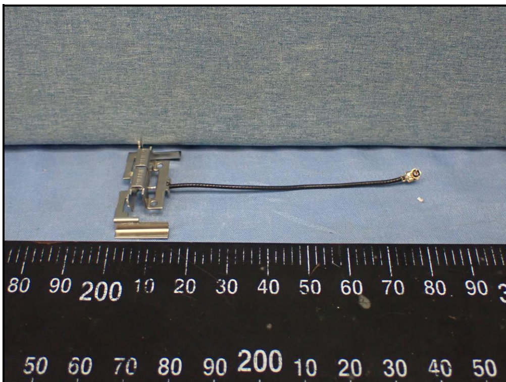
Antenna: 2.4G_0
