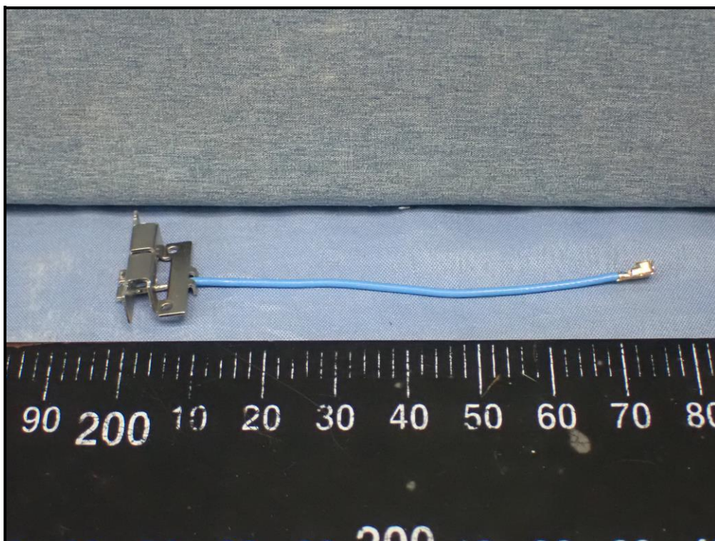
Antenna: 5G_1
