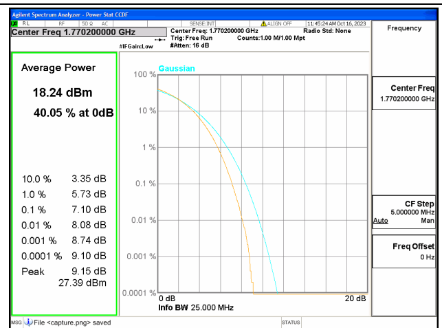
66B / 15+5MHz / High CH / 256QAM
