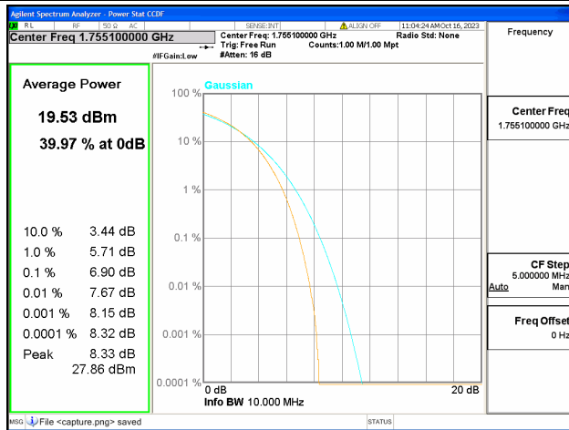
66B / 5+5MHz / Mid CH / 64QAM
