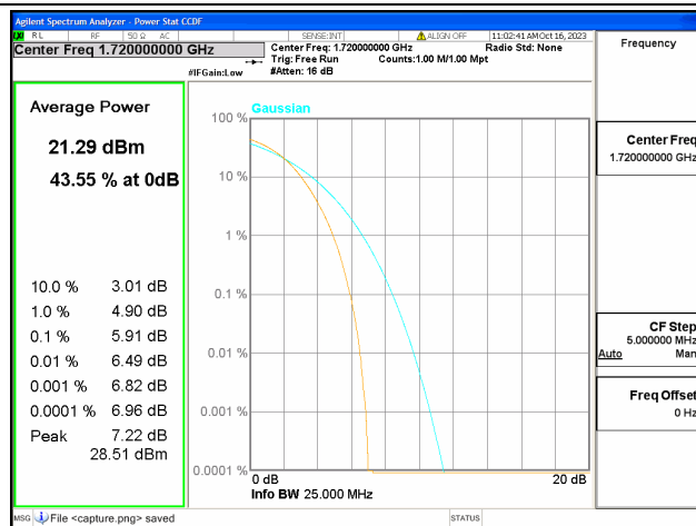
66B / 15+5MHz / Low CH / QPSK
