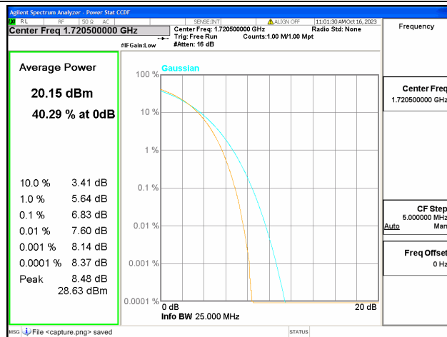
66B / 5+15MHz / Low CH / 64QAM
