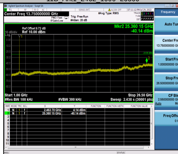
11B_Ant1_2462_1000~26500
