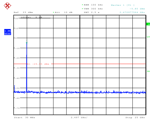
802.11b_2472MHz_Chain 1
