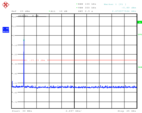
802.11b_2472MHz_Chain 0
