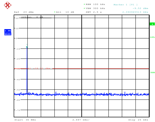
802.11n20_2412MHz_Chain 1
