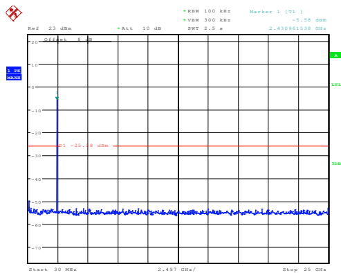
802.11b_2442MHz_Chain 1
