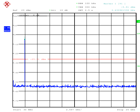
802.11b_2442MHz_Chain 0
