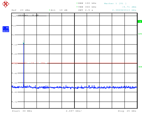
802.11n20_2412MHz_Chain 0
