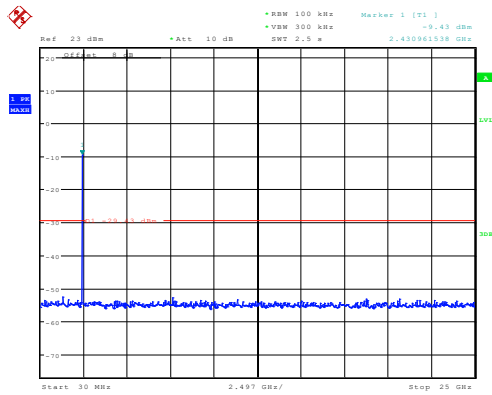
802.11n20_2442MHz_Chain 1
