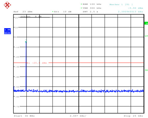
802.11b_2412MHz_Chain 1
