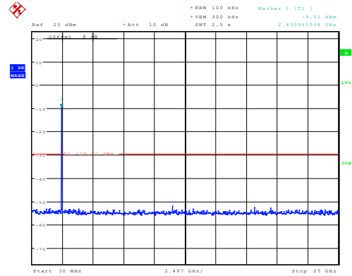
802.11n20_2442MHz_Chain 0
