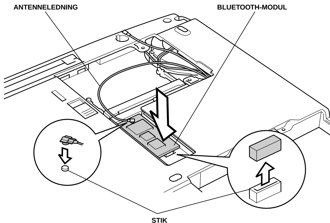
Installation af Bluetooth-modulet
