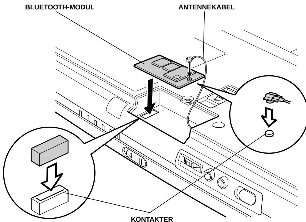
Installere Bluetooth-modulen (Tecra 9000)
