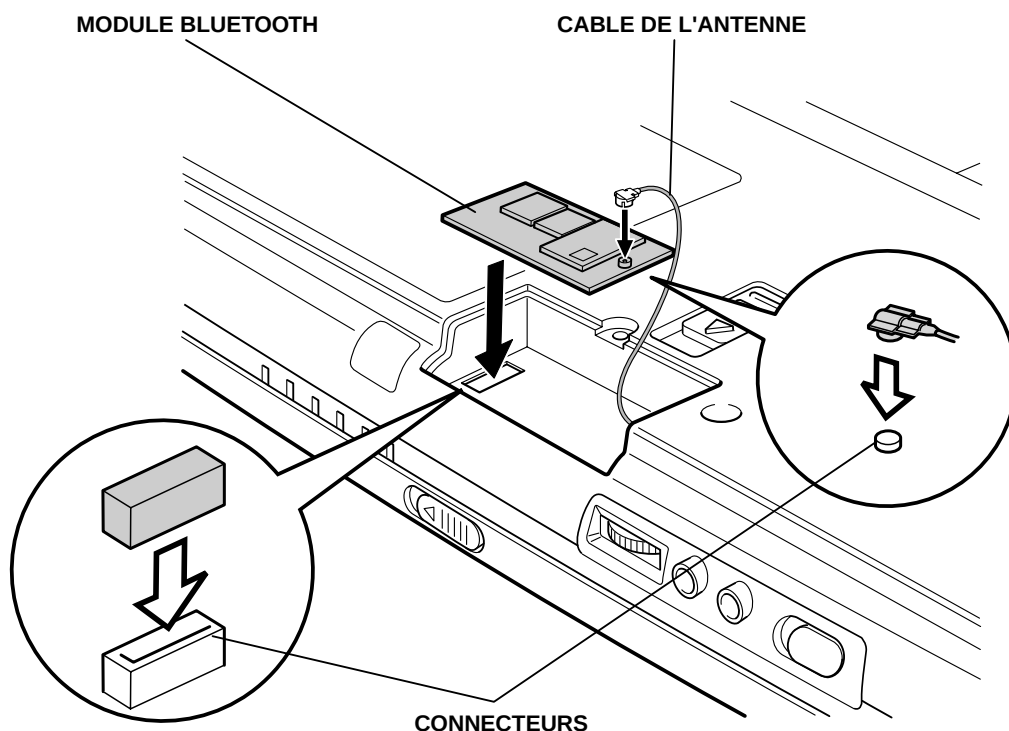
Installation du module Bluetooth (Tecra 9000)
