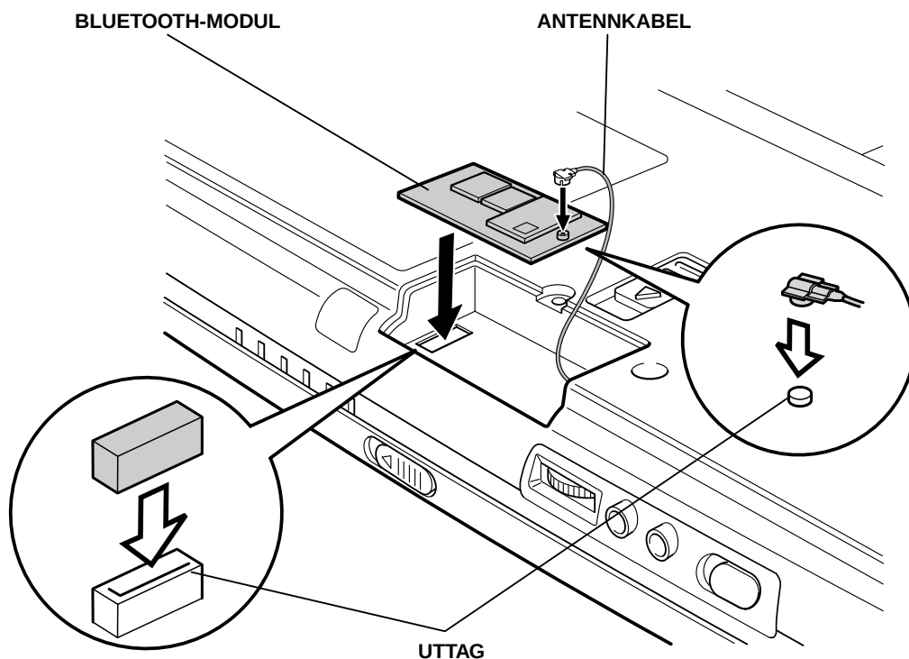
Installera Bluetooth-modulen (Tecra 9000)
