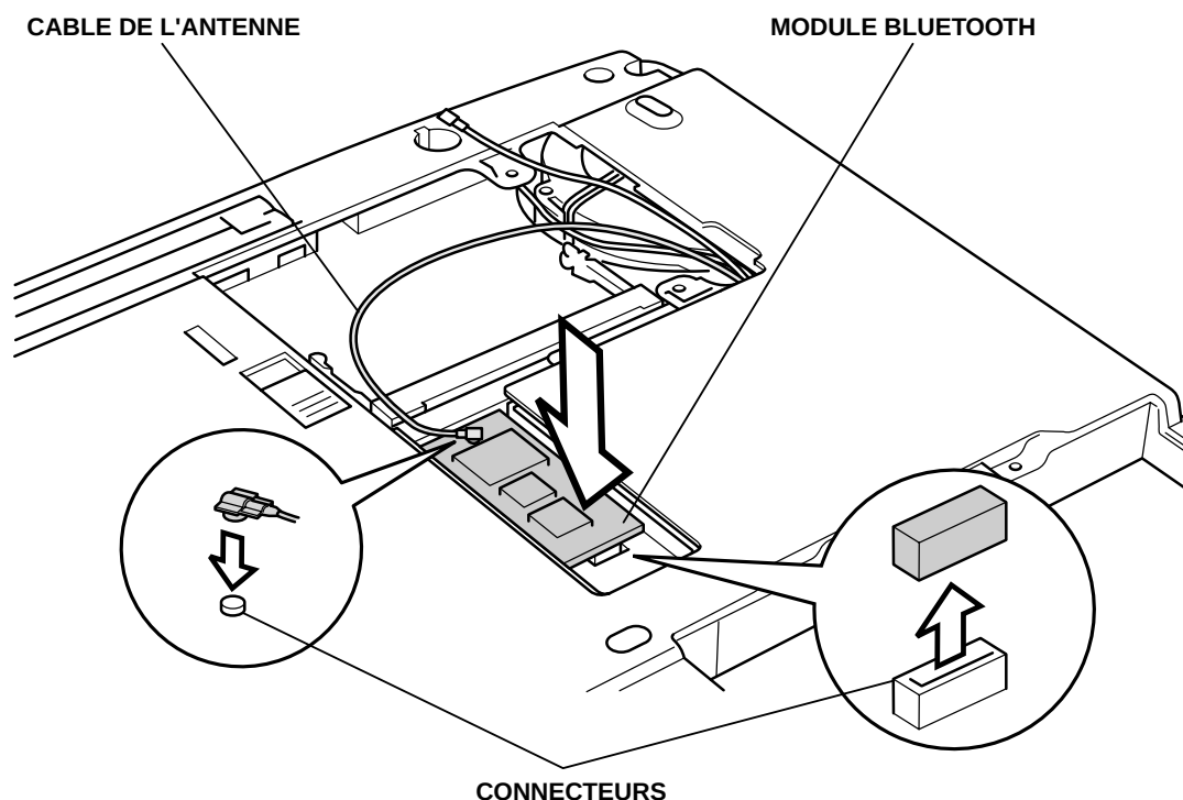
Installation du module Bluetooth
