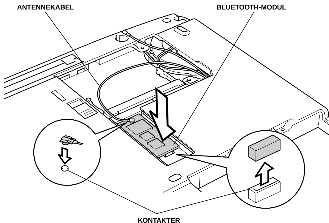
Installere Bluetooth-modulen
