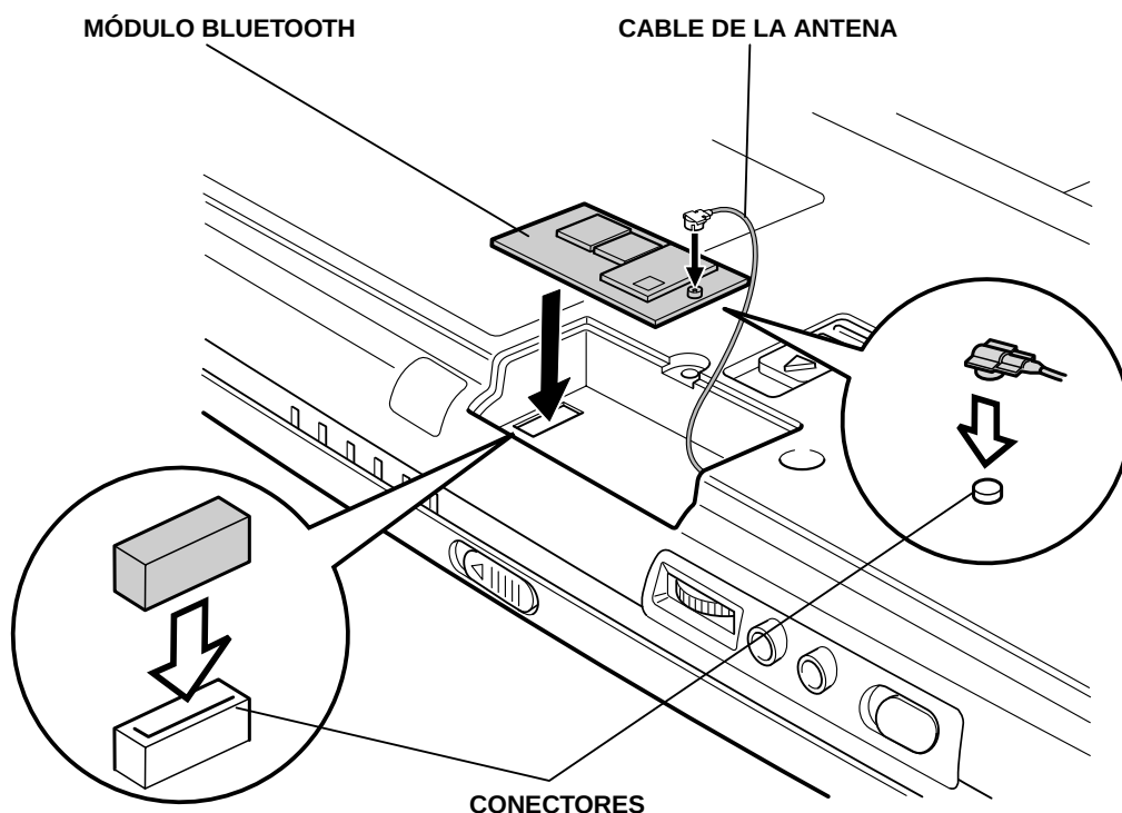
Instalación del módulo Bluetooth (Tecra 9000)
