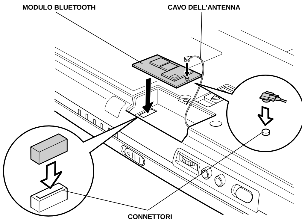
Installazione del modulo Bluetooth (Tecra 9000)
