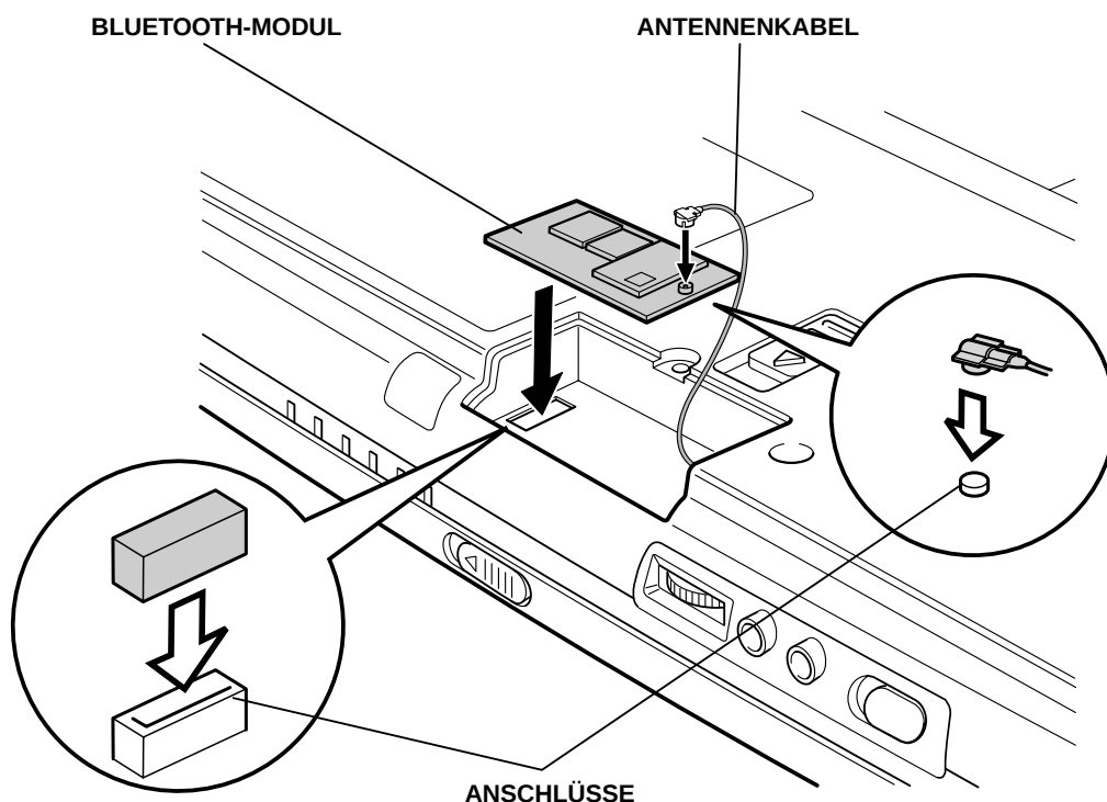
Bluetooth-Modul installieren (Tecra 9000)
