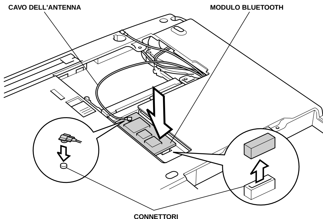
Installazione del modulo Bluetooth
