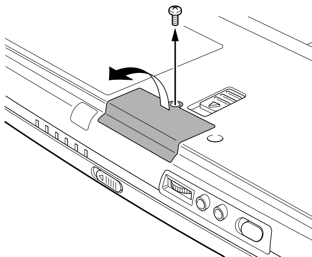
Retrait du capot de l'emplacement Bluetooth
