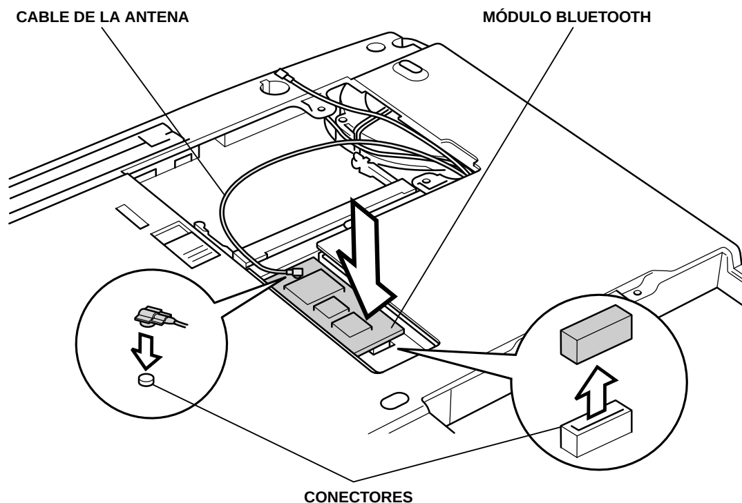
Instalación del módulo Bluetooth
