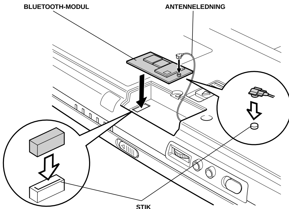
Installation af Bluetooth-modulet (Tecra 9000)
