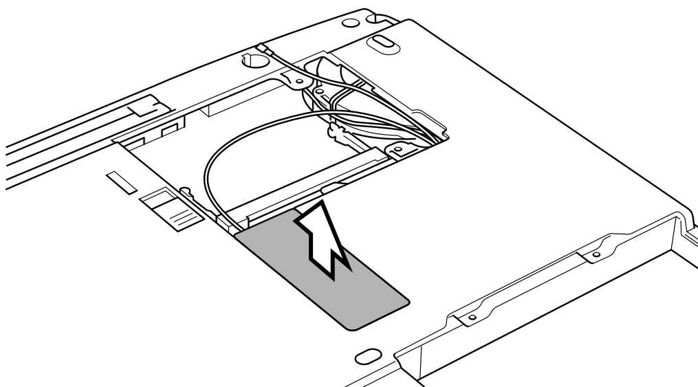
Fjerne spordekslet for Bluetooth-modulen
