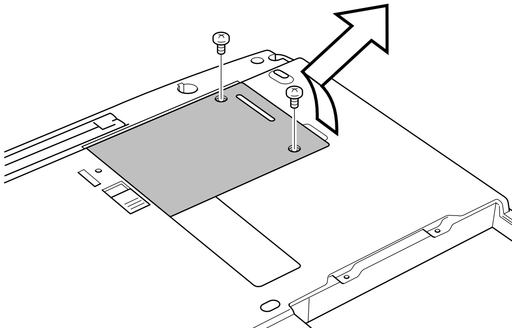
Abdeckung über dem Wireless LAN Card-Steckplatz entfernen
