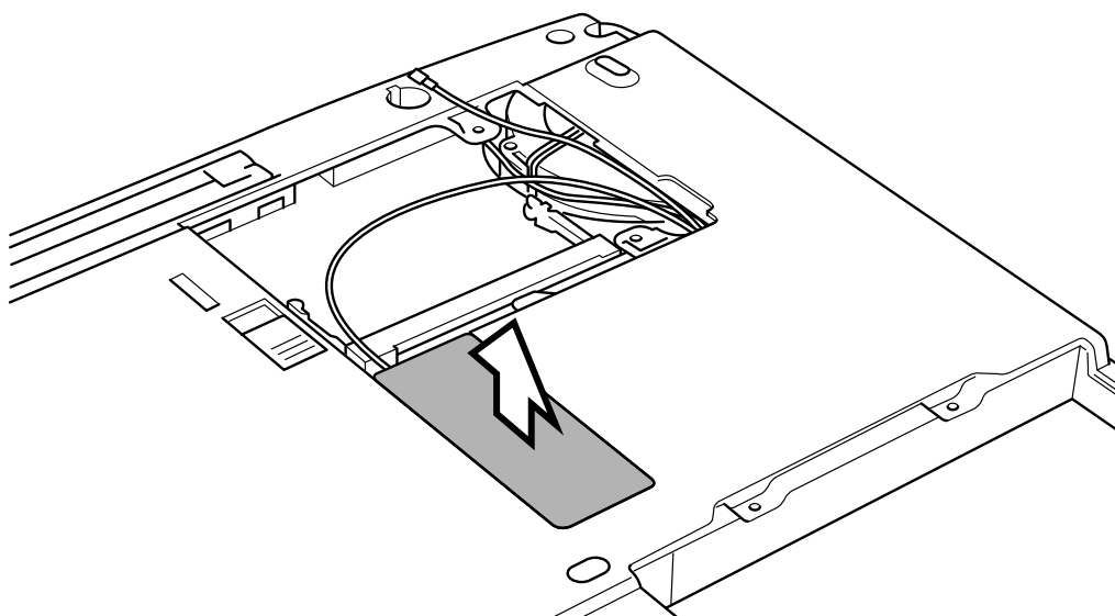
Abdeckung über dem Bluetooth-Modulsteckplatz entfernen
