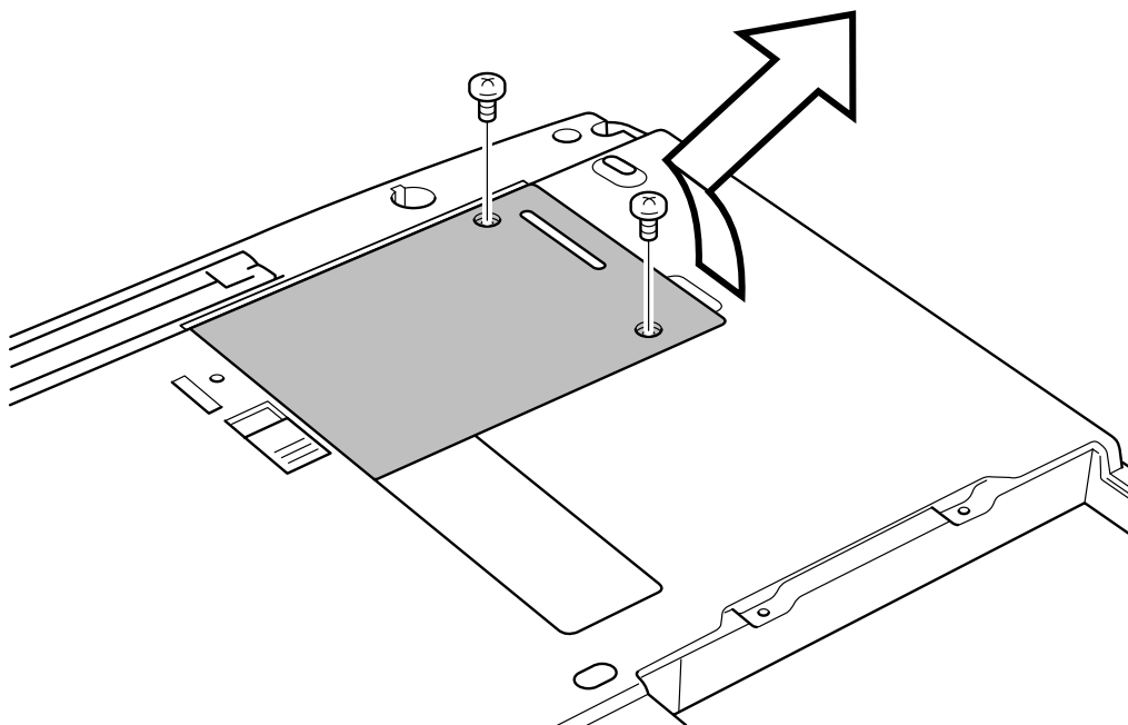
Løfte spordekslet for Bluetooth-modulen
