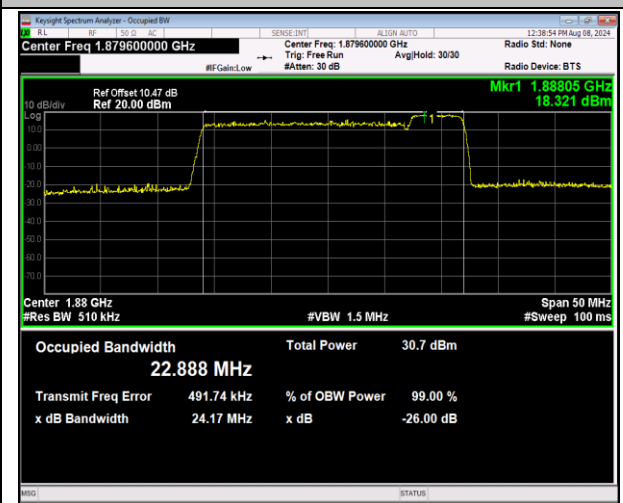
2-2-20MHz-5MHz-QPSK-QPSK-18875-18992-100RB#0-25RB#0-PASS
