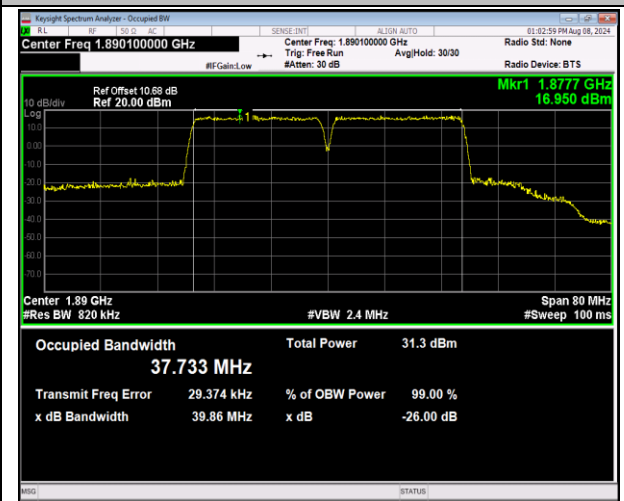
2-2-20MHz-20MHz-QPSK-QPSK-18902-19100-100RB#0-100RB#0-PASS
