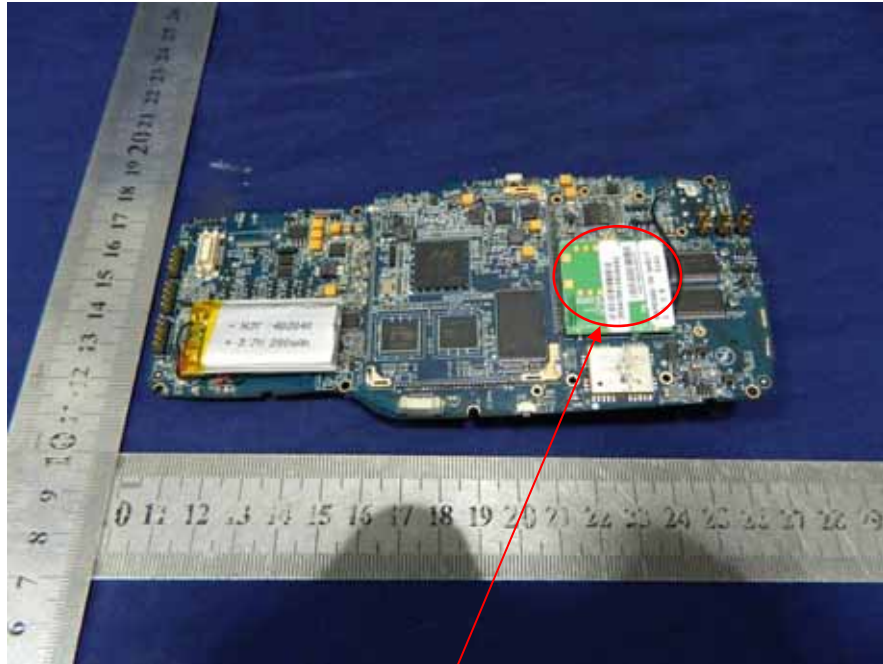
2G Module
