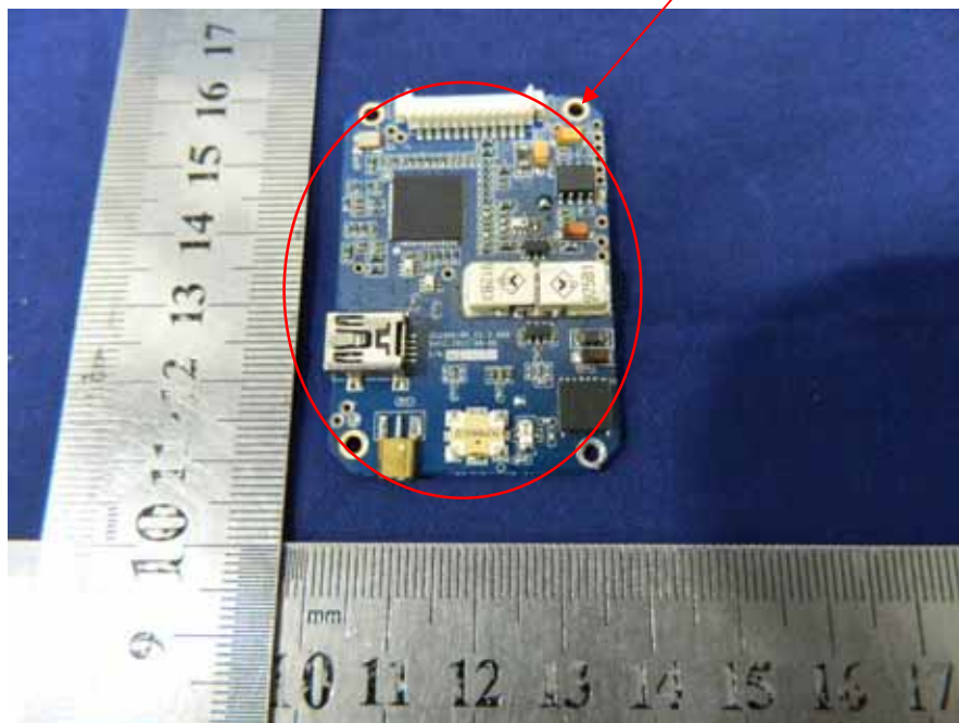
RFID module
