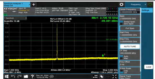
Band25-3MHz-QPSK-26365-1RB#0-1000~3000-PASS
