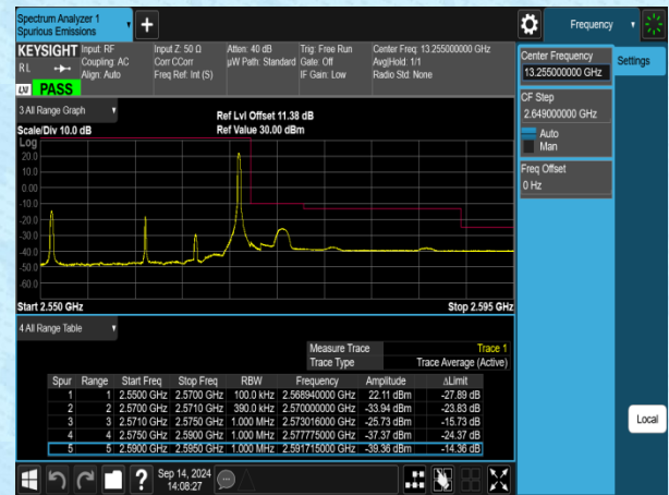
Band7-20MHz-QPSK-21350-1RB#99-PASS
