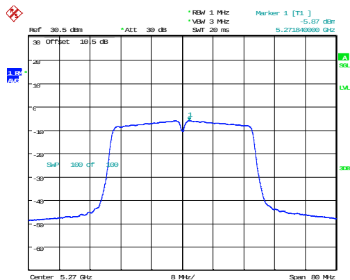
802.11n40_5270MHz
