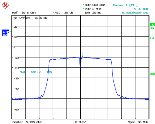
802.11n40_5795MHz
