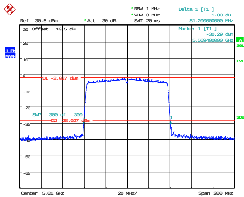
802.11ac80_5610MHz
