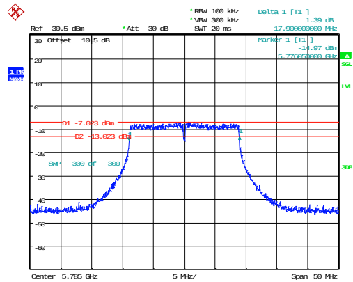
802.11n20_5785MHz
