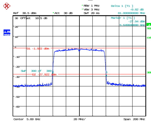
802.11ac80_5690MHz
