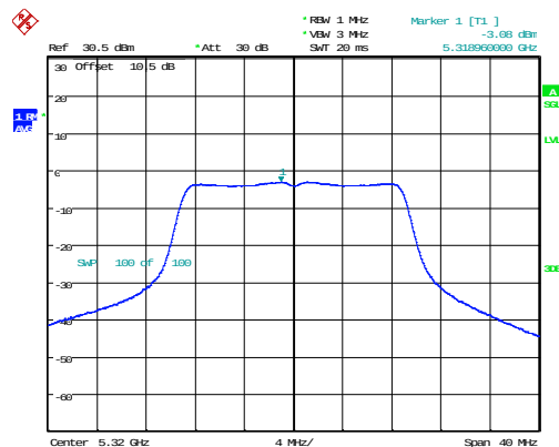
802.11n20_5320MHz
