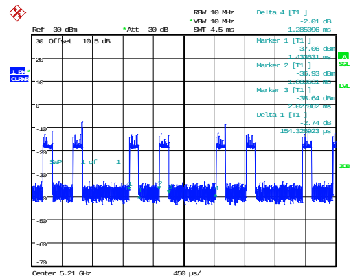
802.11ax80_5210MHz_RU_242/61
