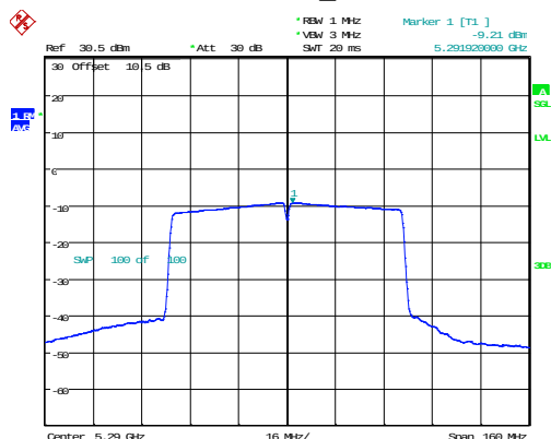
802.11ac80_5290MHz
