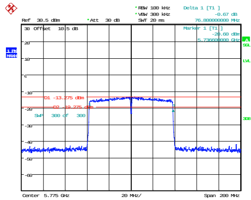
802.11ac80_5775MHz
