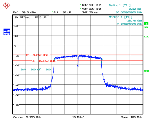
802.11n40_5755MHz
