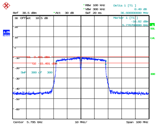
802.11n40_5795MHz
