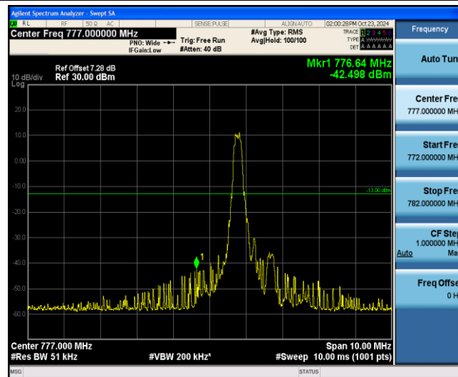
Band13-10MHz-QPSK-23230-1-0-Low--42.50-PASS
