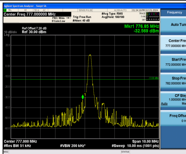
Band13-5MHz-QPSK-23205-1-0-Low--32.57-PASS
