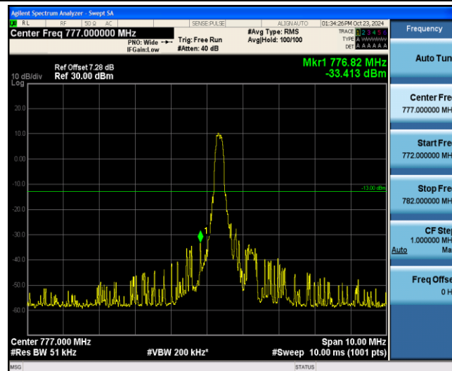
Band13-5MHz-16QAM-23205-1-0-Low--33.41-PASS
