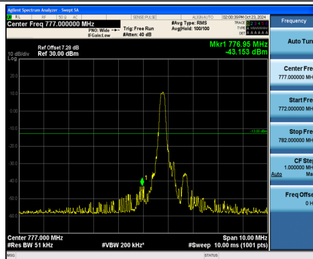
Band13-10MHz-16QAM-23230-1-0-Low--43.15-PASS
