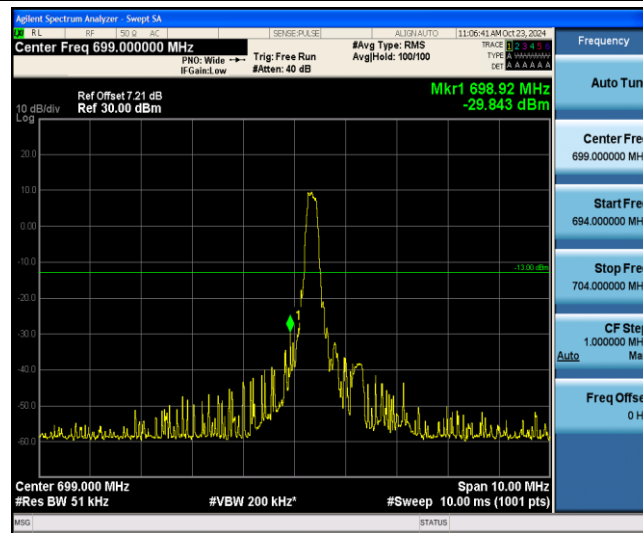
Band12-5MHz-QPSK-23035-1-0-Low--29.84-PASS
