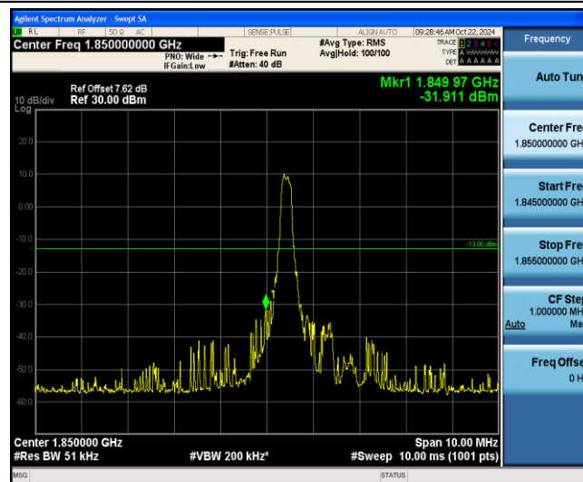
Band2-3MHz-QPSK-18615-1-0-Low--31.91-PASS
