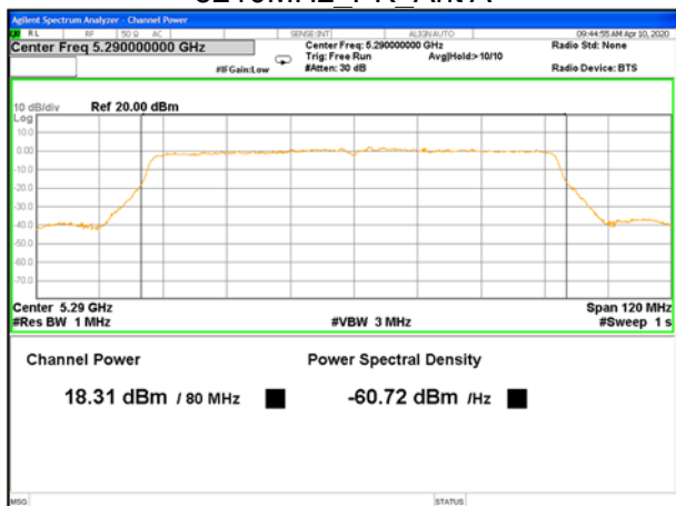
5290MHz_PK_Ant A
