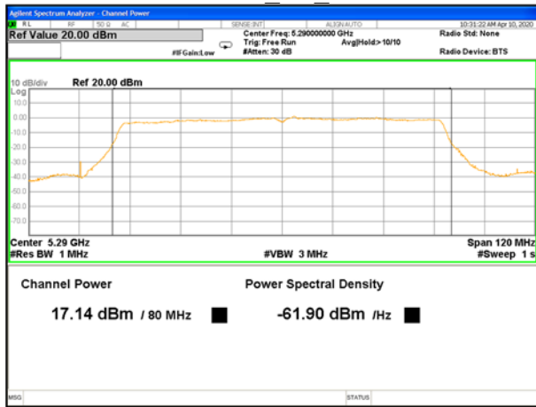
5290MHz_PK_Ant B
