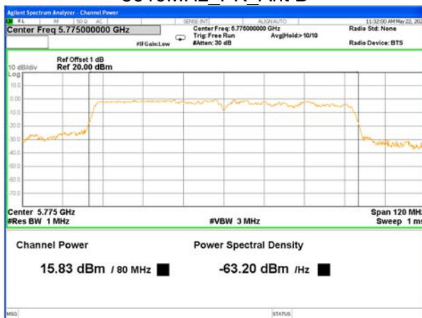
5775MHz_PK_Ant B
