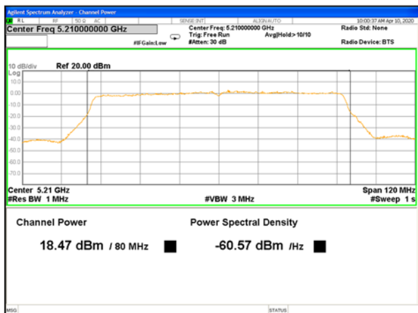
5210MHz_PK_Ant A
