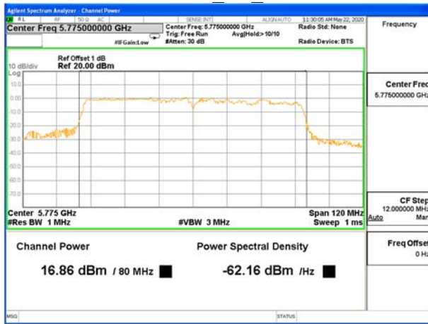
5775MHz_PK_Ant A
