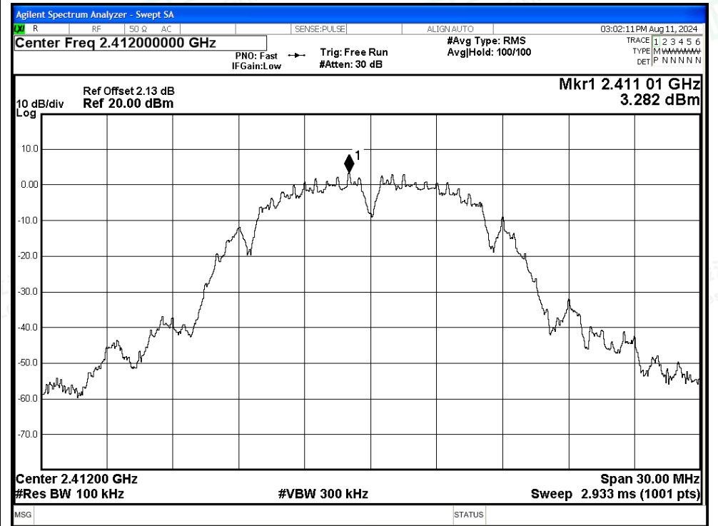
Band Edge NVNT b 2412MHz Ant Emission
