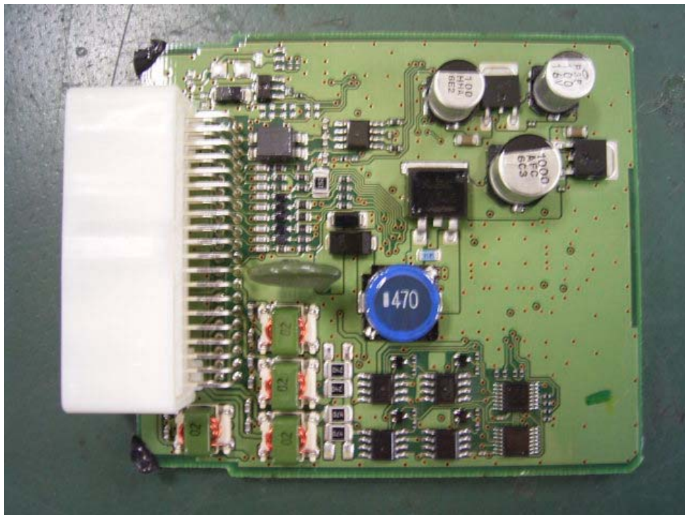
PCB Top
