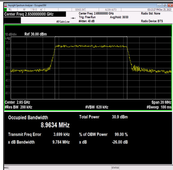
41(2535-2655)-10MHz-64QAM-41190-50RB#0-PASS
