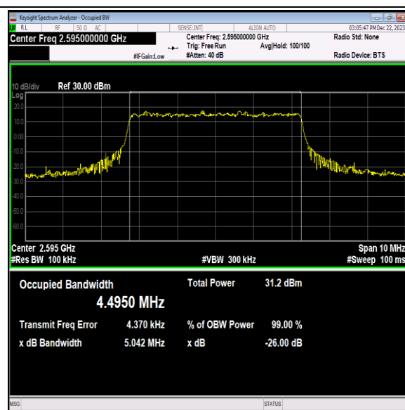
41(2535-2655)-5MHz-64QAM-40640-25RB#0-PASS
