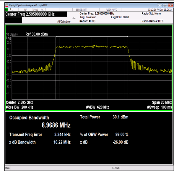
41(2535-2655)-10MHz-16QAM-40640-50RB#0-PASS
