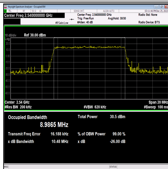
41(2535-2655)-10MHz-QPSK-40090-50RB#0-PASS
