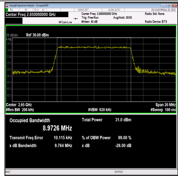
41(2535-2655)-10MHz-QPSK-41190-50RB#0-PASS
