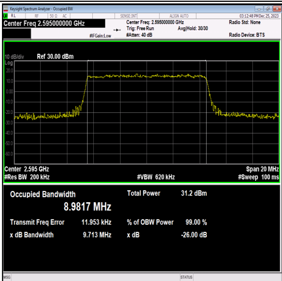
41(2535-2655)-10MHz-64QAM-40640-50RB#0-PASS
