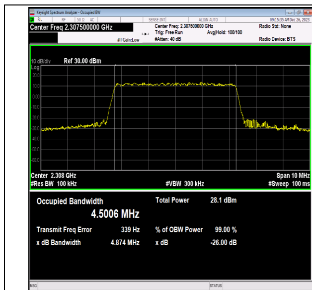
40(2305-2315)-5MHz-64QAM-38725-25RB#0-PASS
