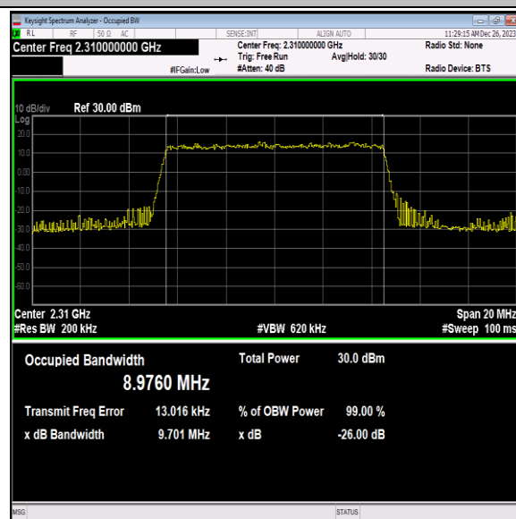
40(2305-2315)-10MHz-QPSK-38750-50RB#0-PASS
