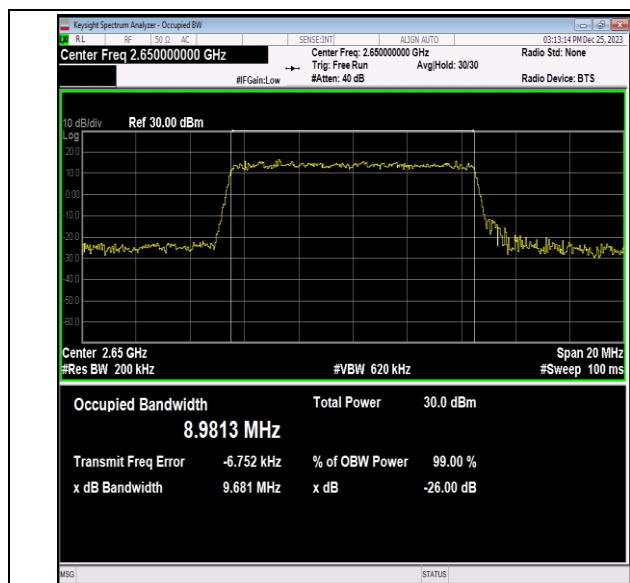
41(2535-2655)-10MHz-16QAM-41190-50RB#0-PASS
