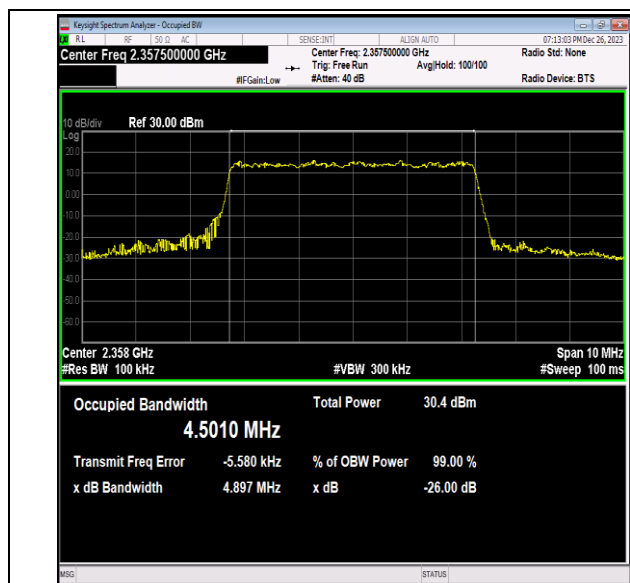
40(2350-2360)-5MHz-QPSK-39225-25RB#0-PASS
