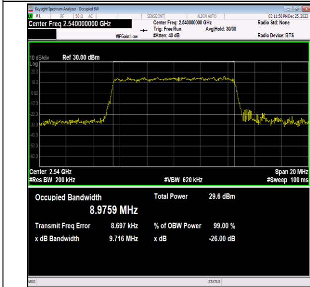
41(2535-2655)-10MHz-16QAM-40090-50RB#0-PASS
