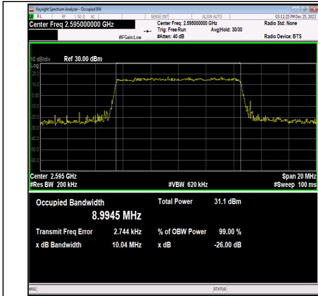
41(2535-2655)-10MHz-QPSK-40640-50RB#0-PASS
