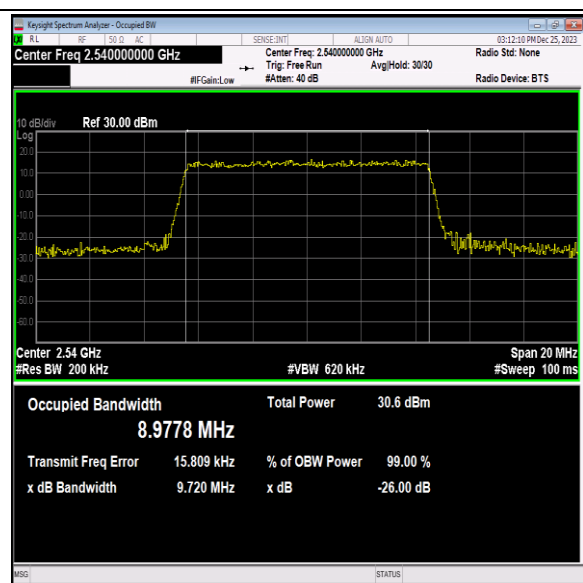
41(2535-2655)-10MHz-64QAM-40090-50RB#0-PASS
