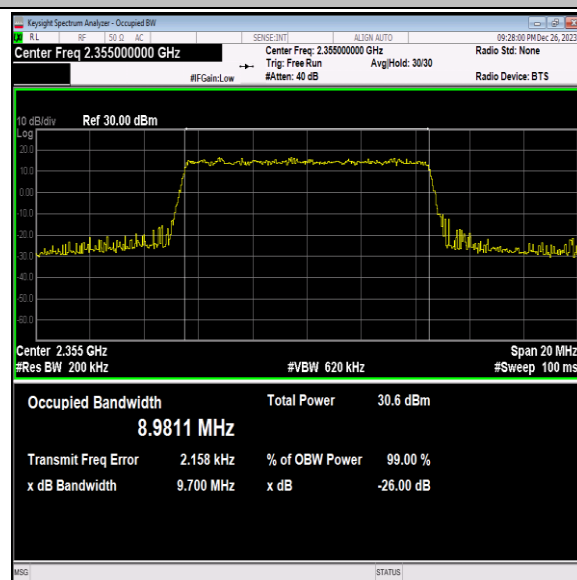
40(2350-2360)-10MHz-QPSK-39200-50RB#0-PASS
