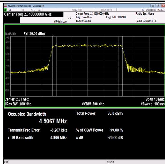
40(2305-2315)-5MHz-QPSK-38750-25RB#0-PASS
