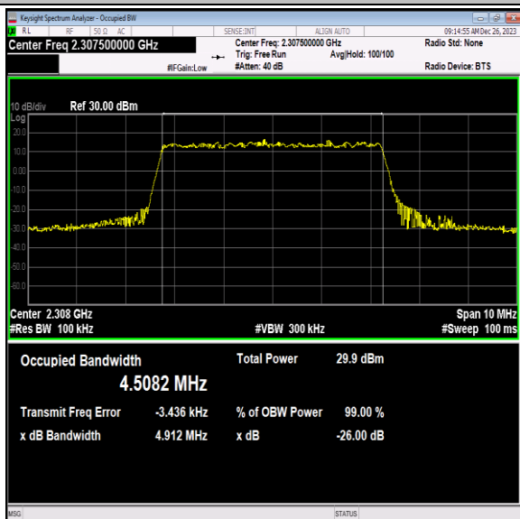
40(2305-2315)-5MHz-QPSK-38725-25RB#0-PASS
