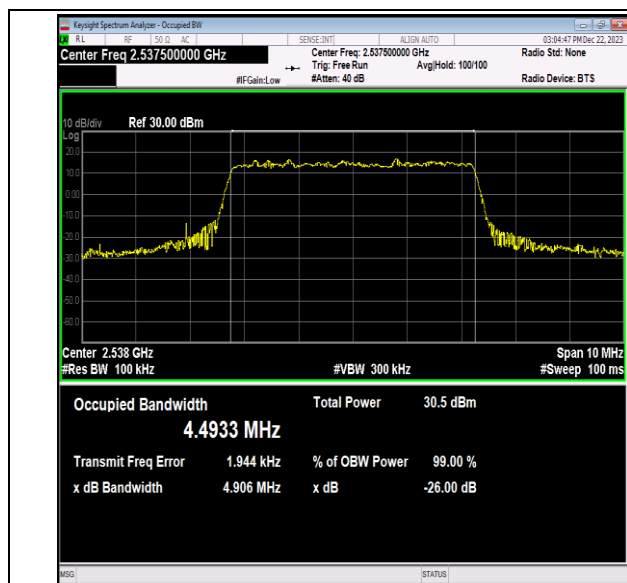
41(2535-2655)-5MHz-64QAM-40065-25RB#0-PASS
