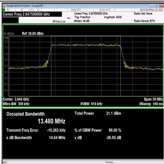
41(2535-2655)-15MHz-QPSK-41165-75RB#0-PASS
