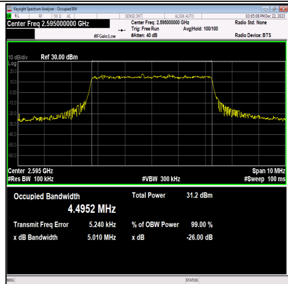
41(2535-2655)-5MHz-QPSK-40640-25RB#0-PASS
