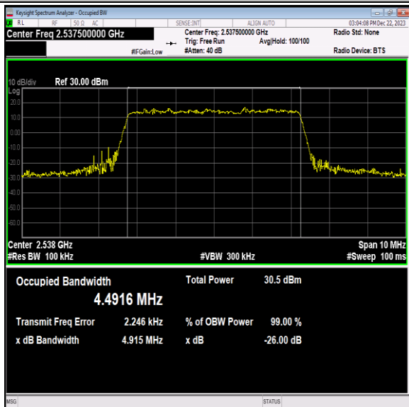
41(2535-2655)-5MHz-QPSK-40065-25RB#0-PASS
