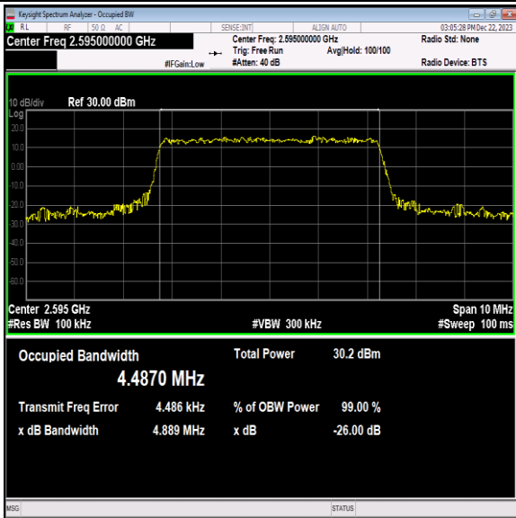
41(2535-2655)-5MHz-16QAM-40640-25RB#0-PASS
