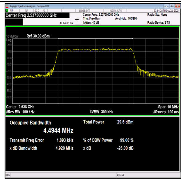
41(2535-2655)-5MHz-16QAM-40065-25RB#0-PASS
