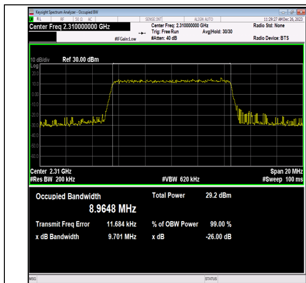
40(2305-2315)-10MHz-16QAM-38750-50RB#0-PASS
