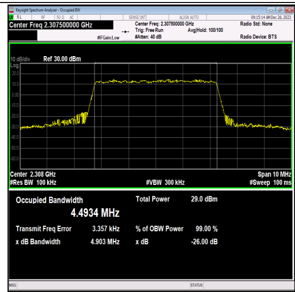
40(2305-2315)-5MHz-16QAM-38725-25RB#0-PASS
