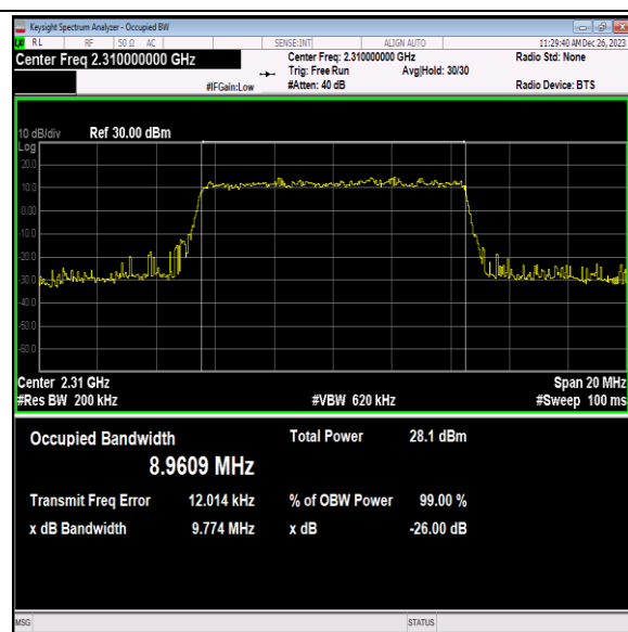
40(2305-2315)-10MHz-64QAM-38750-50RB#0-PASS
