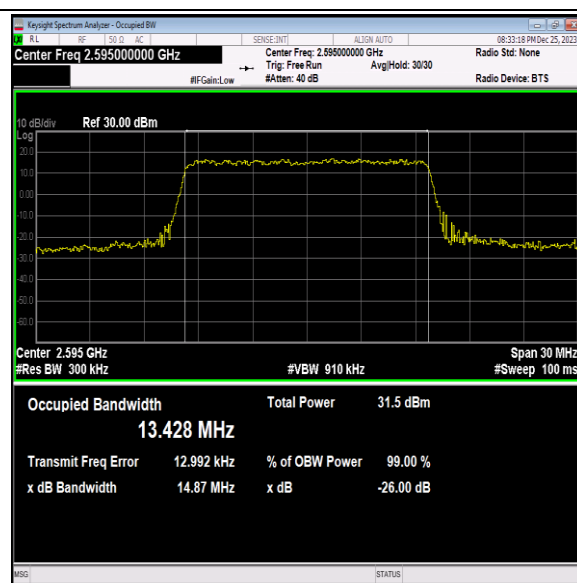
41(2535-2655)-15MHz-QPSK-40640-75RB#0-PASS
