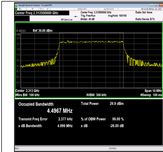
40(2305-2315)-5MHz-QPSK-38775-25RB#0-PASS
