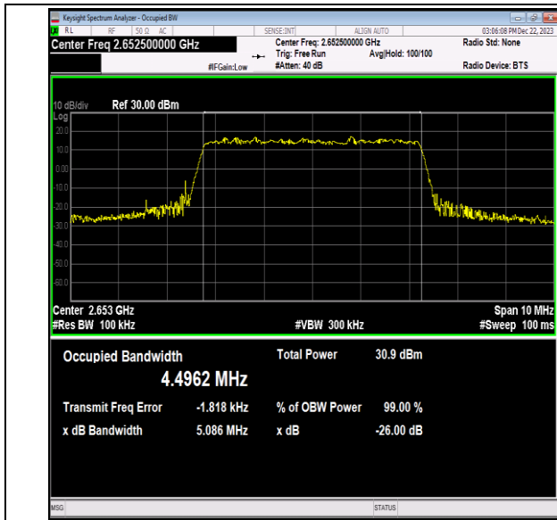
41(2535-2655)-5MHz-QPSK-41215-25RB#0-PASS
