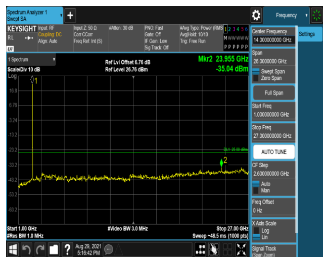
Band38-20MHz-QPSK-38150:1000~27000MHz
