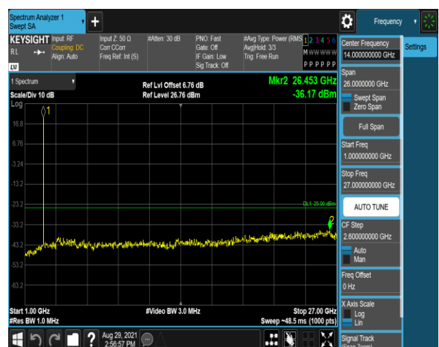
Band7-5MHz-16QAM-21425:1000~27000MHz
