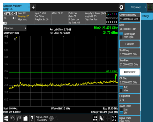
Band7-5MHz-QPSK-21425:1000~27000MHz
