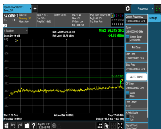
Band7-20MHz-QPSK-21350:1000~27000MHz
