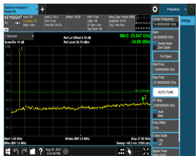
Band41-5MHz-QPSK-41215:1000~27000MHz
