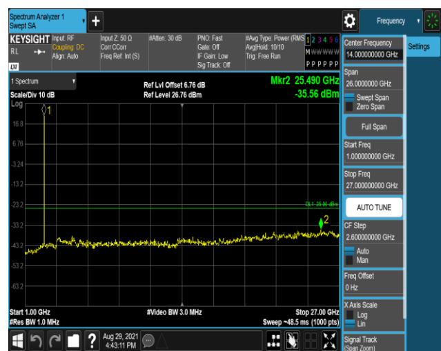
Band38-5MHz-QPSK-38225:1000~27000MHz
