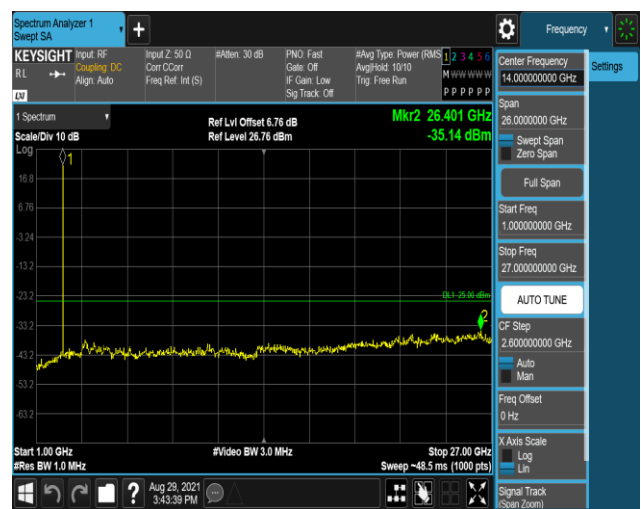
Band41-5MHz-QPSK-40640:1000~27000MHz
