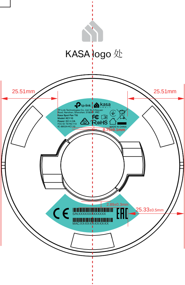
尺寸图
