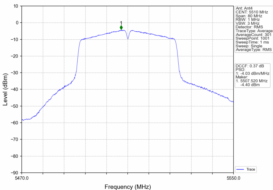
802.11n(HT40)_LCH_5510MHz_Ant4_NTNV
